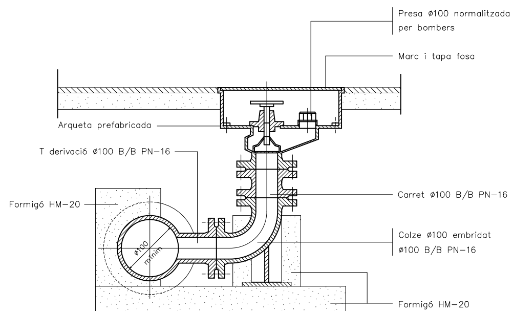
DETALL D'ESCOMESA DOMICILIÀRIA ESCALA S/E
