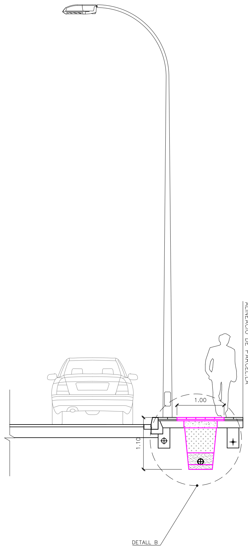
SECCIÓ DETALL DE RASA EN VORERA ESCALA 1/50
