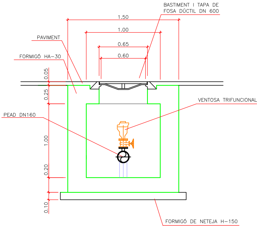
SECCIÓ A-A' ESCALA 1:40
