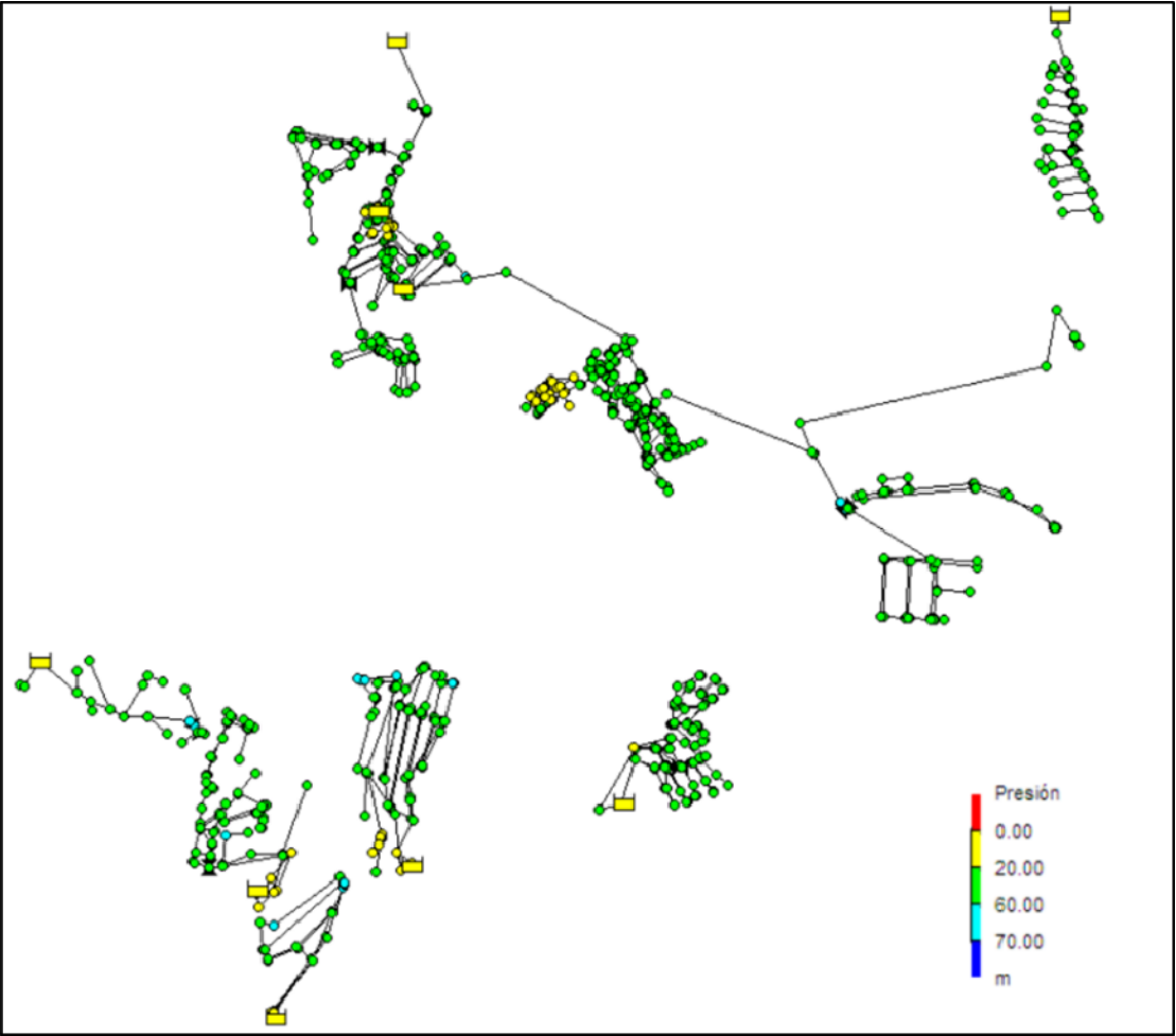
Imatge 1. Distribució general de les pressions segons modelització (en m.c.m.)
