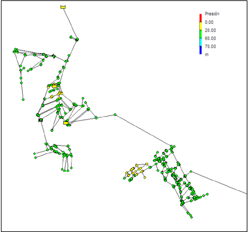
Imatge 2. Distribució de pressions a la xarxa del poble i el priorat segons modelització (en m.c.m.)
