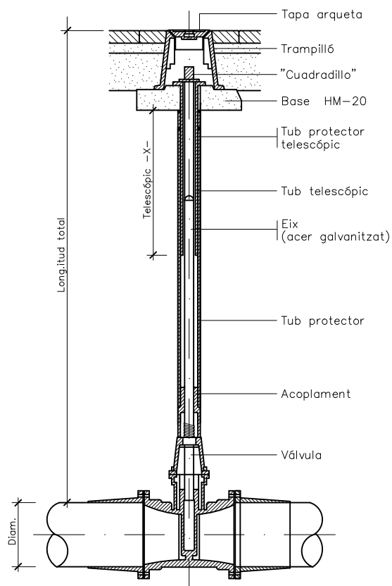
DETALL DE VÀLVULA DE COMPORTA I EIX TELESCÒPIC ESCALA S/E
