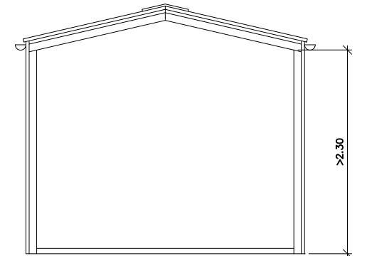
SECCIÓ A-B
