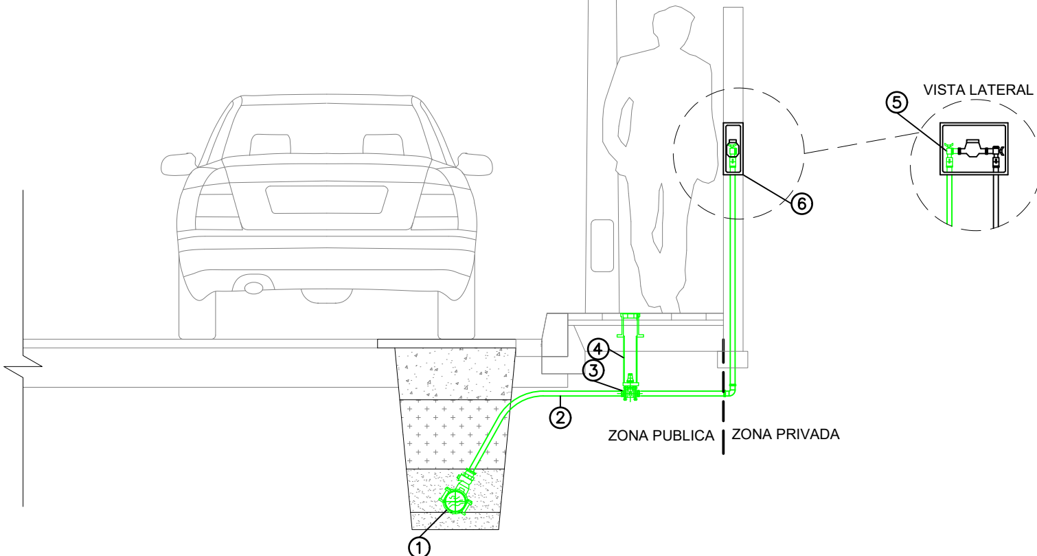
DETALL D'ESCOMESA DOMICILIÀRIA ESCALA S/E
