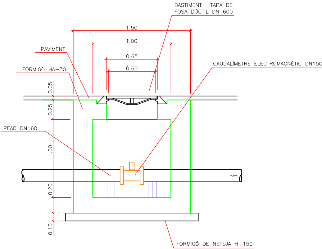
SECCIÓ A-A' ESCALA 1:40
