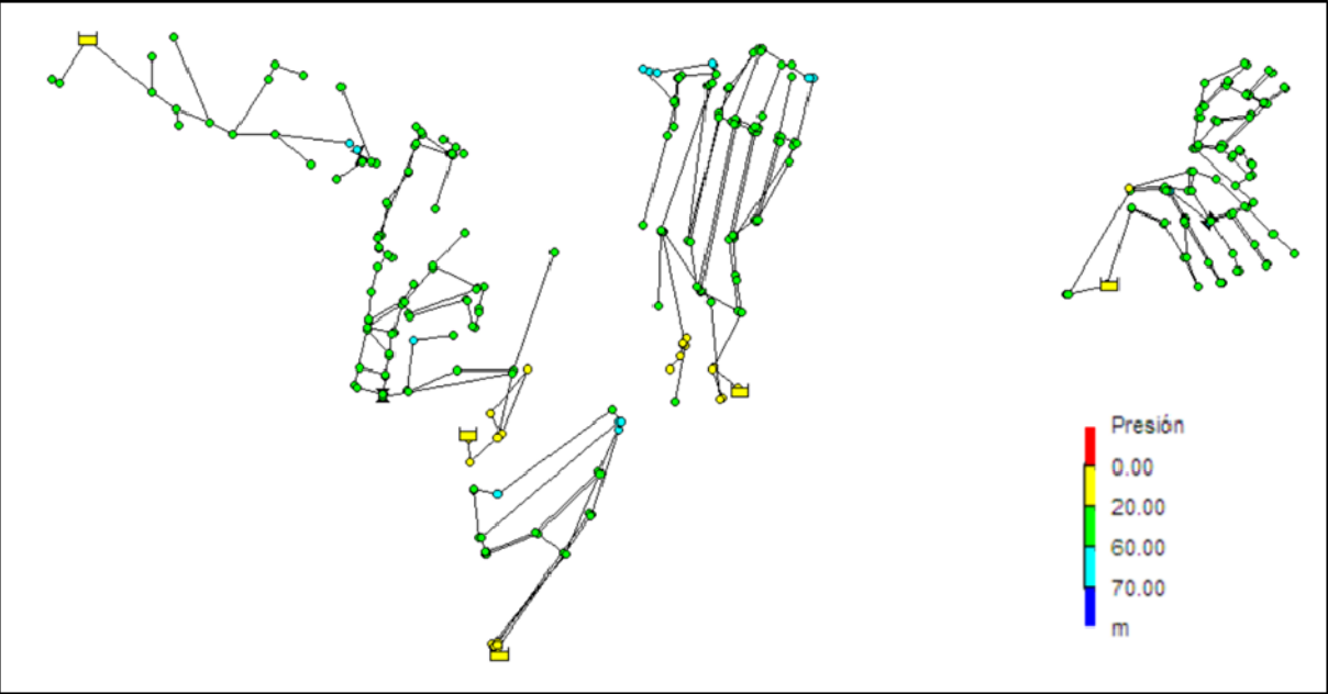
Imatge Error! No hi ha text de l'estil especificat en el document.-1. Distribució de pressions a la xarxa de la Miralba, Can Gordei 1 i 2, l'Esplai i la Masieta segons modelització (en m.c.m.)
