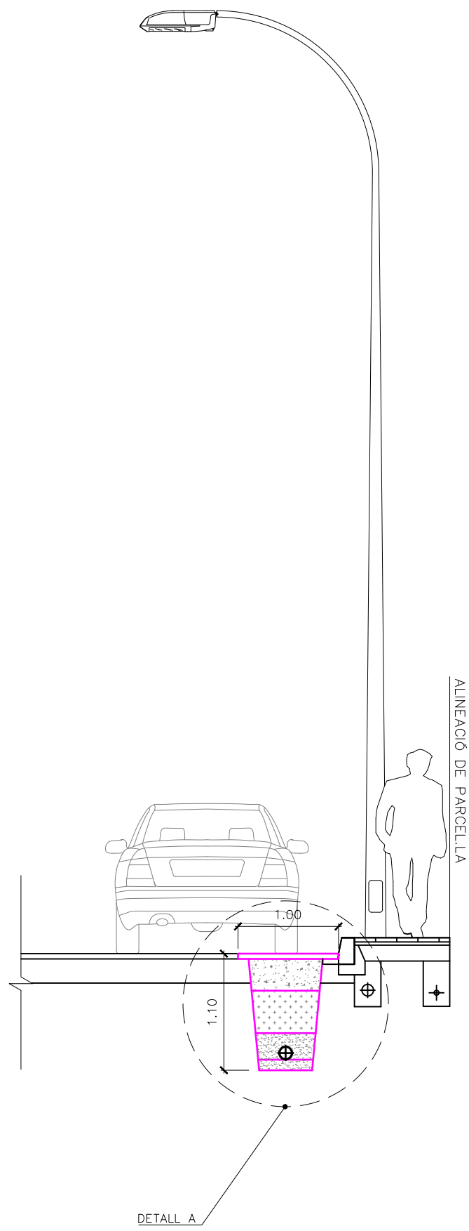
SECCIÓ DETALL DE RASA EN CALÇADA ESCALA 1/50
