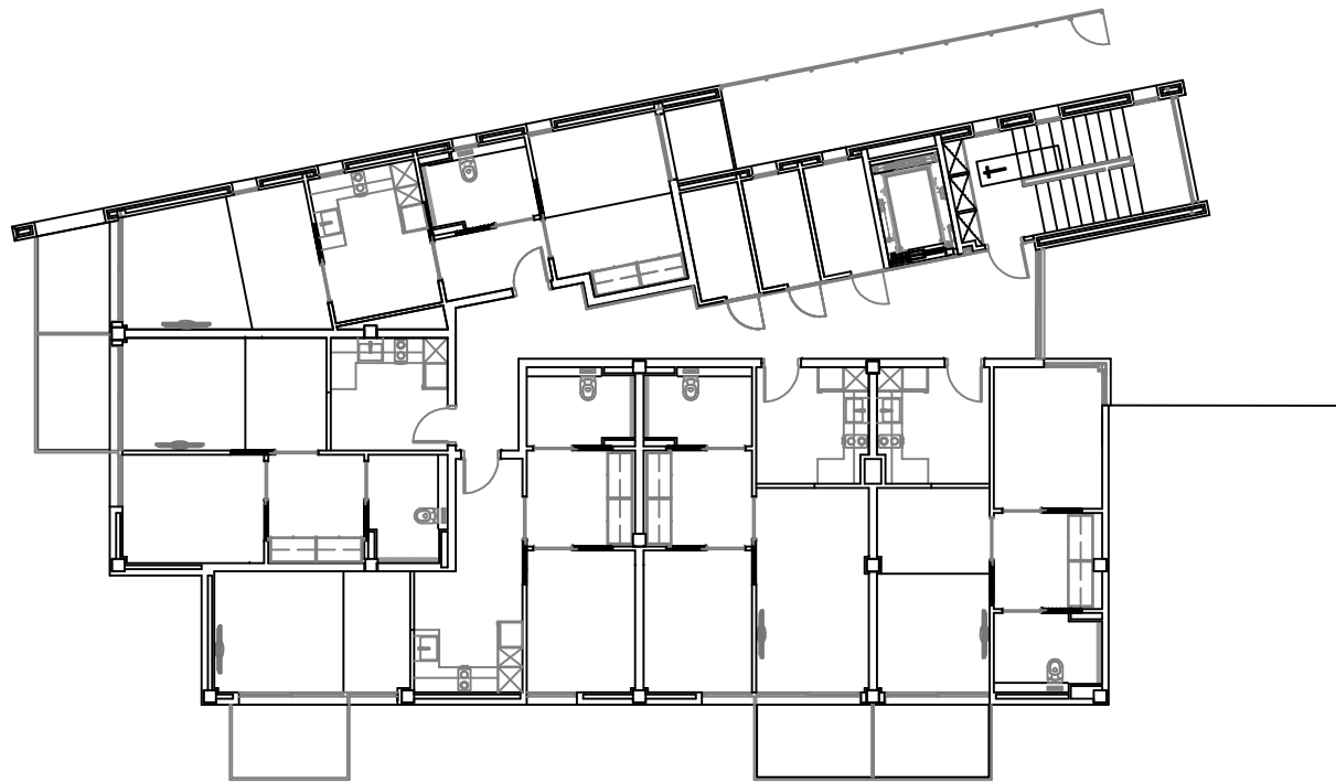
PLANTES PRIMERA, SEGONA I TERCERA
