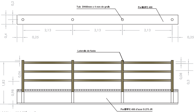
DETALL PASSERA - SECCIÓ A-A'
