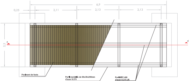
DETALL PASSERA - PLANTA
