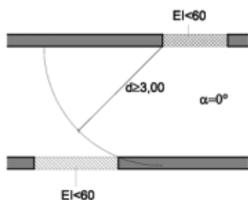
Figura 1.1. Fachadas enfrentadas
