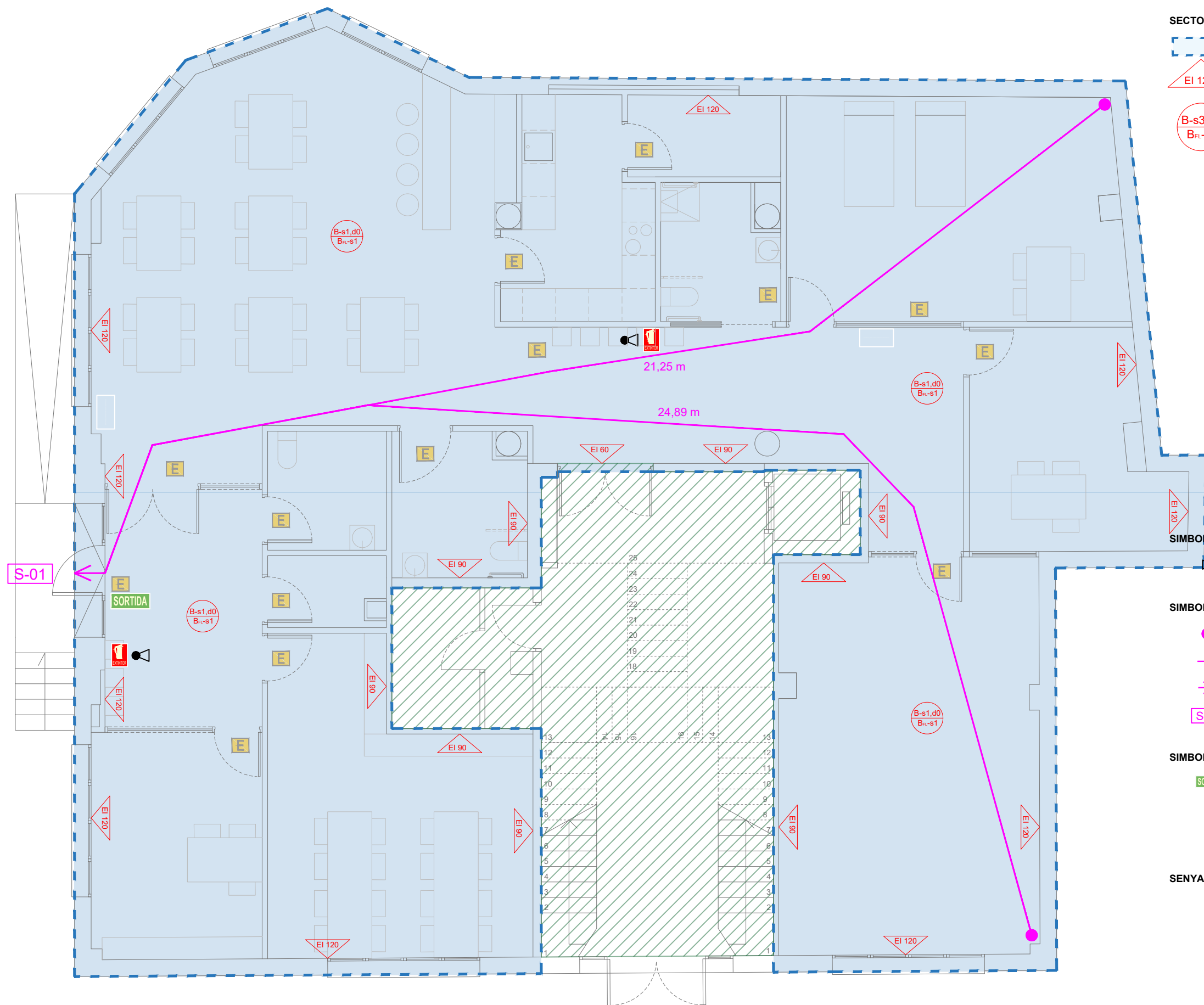
PLANTA BAIXA - INSTAL·LACIÓ PROTECCIÓ CONTRA INCENDIS E1:75 ZONA SENSE ACTUACIÓ
