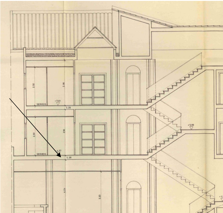
Secció edifici projecte original – característiques forjat p1 (sostre PB)
