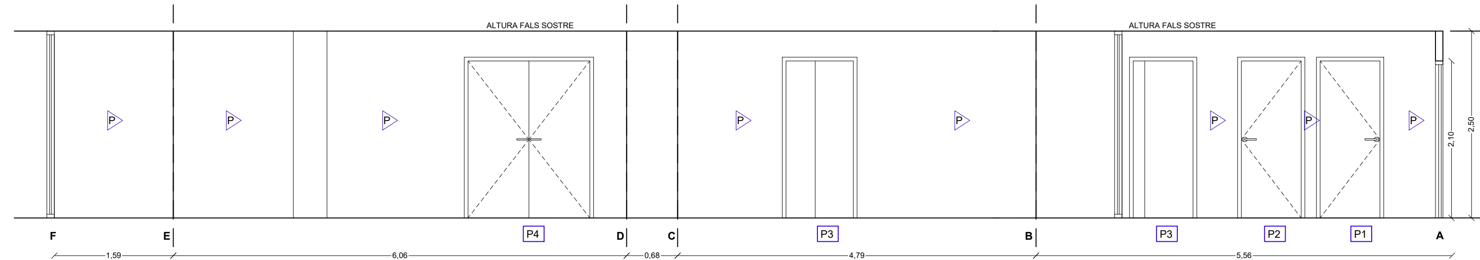
DESPLEGAT ALÇAT FRONTAL PARET ESPERA-DISTRIBUÏDOR E1:50
