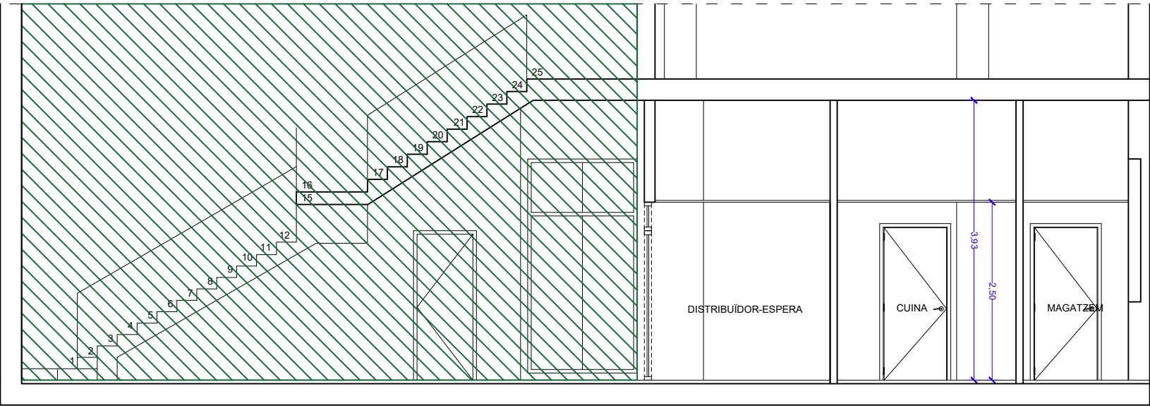
SECCIÓ A2 - PROPOSTA E1:75
