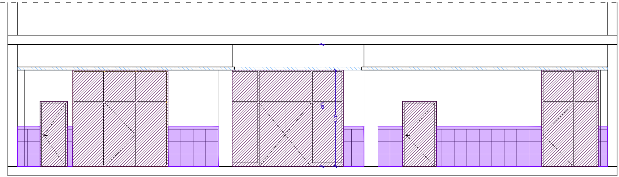
SECCIÓ 1 - ENDERROCS E1:75
