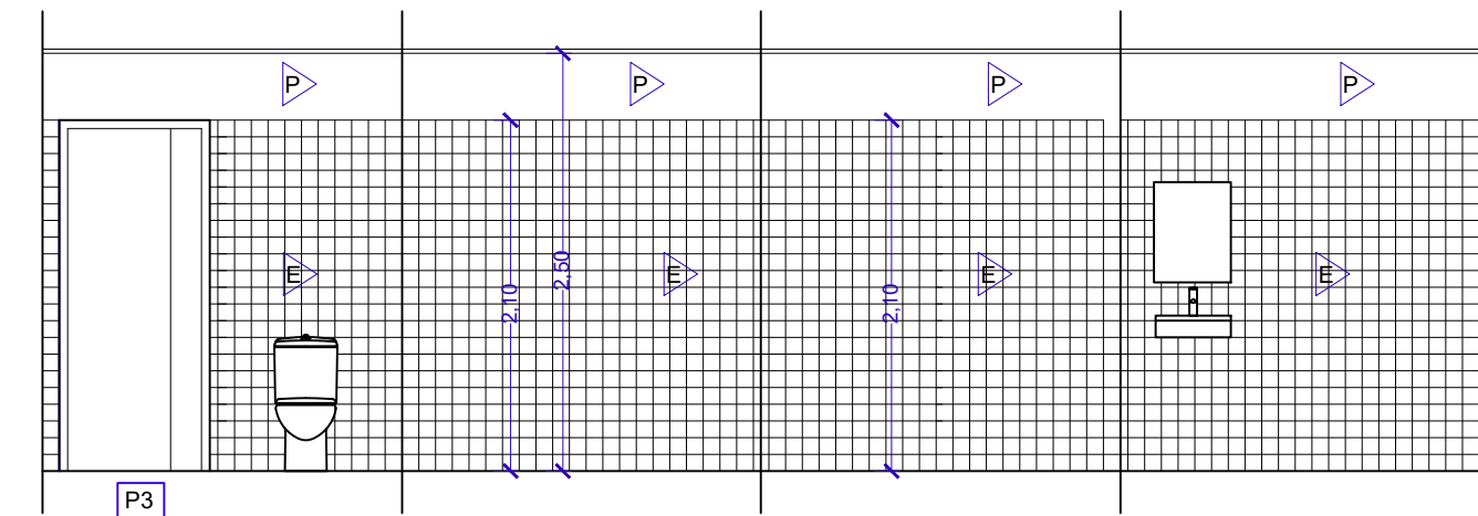
DESPLEGAT ACABATS BANY TIPUS E1:50
