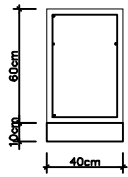
SABATA 40x60 40x60 arm. superior 3ø16, arm. inferior 3ø16, 4ø12 de pell, 1ø4Rø8c/25. 10cm de formigó de neteja
