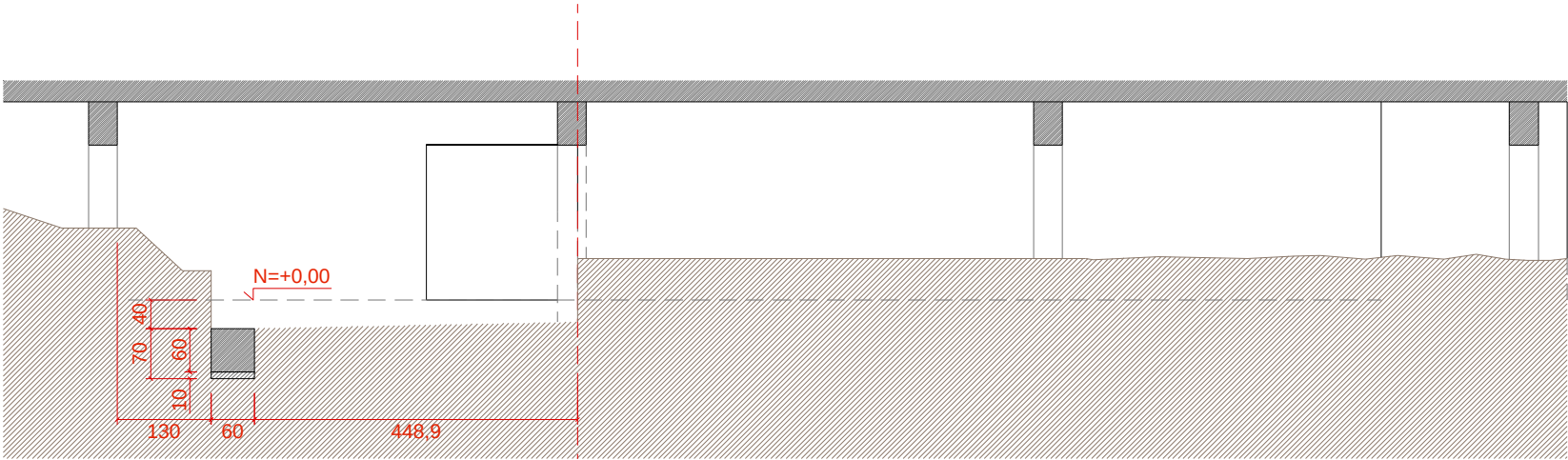
SECCIÓ A
