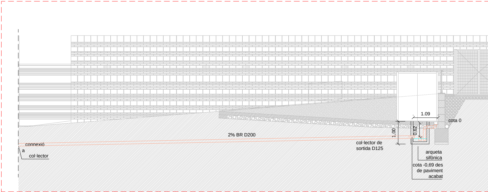
Secció a-a' e: 1/120
