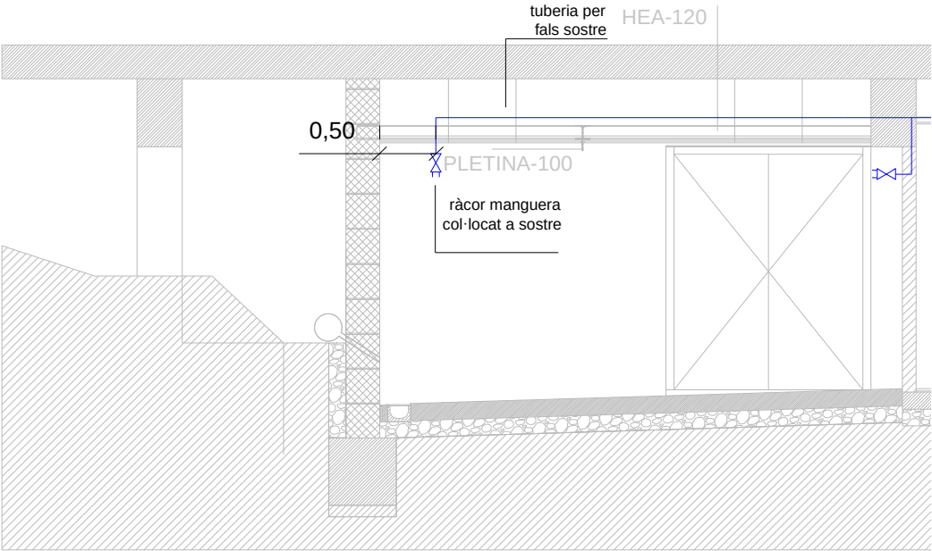
secció b-b'
