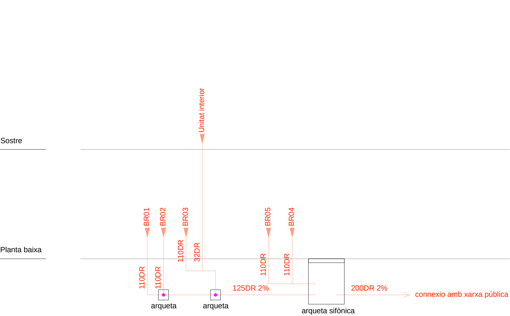
Esquema desguàs aigües residuals
