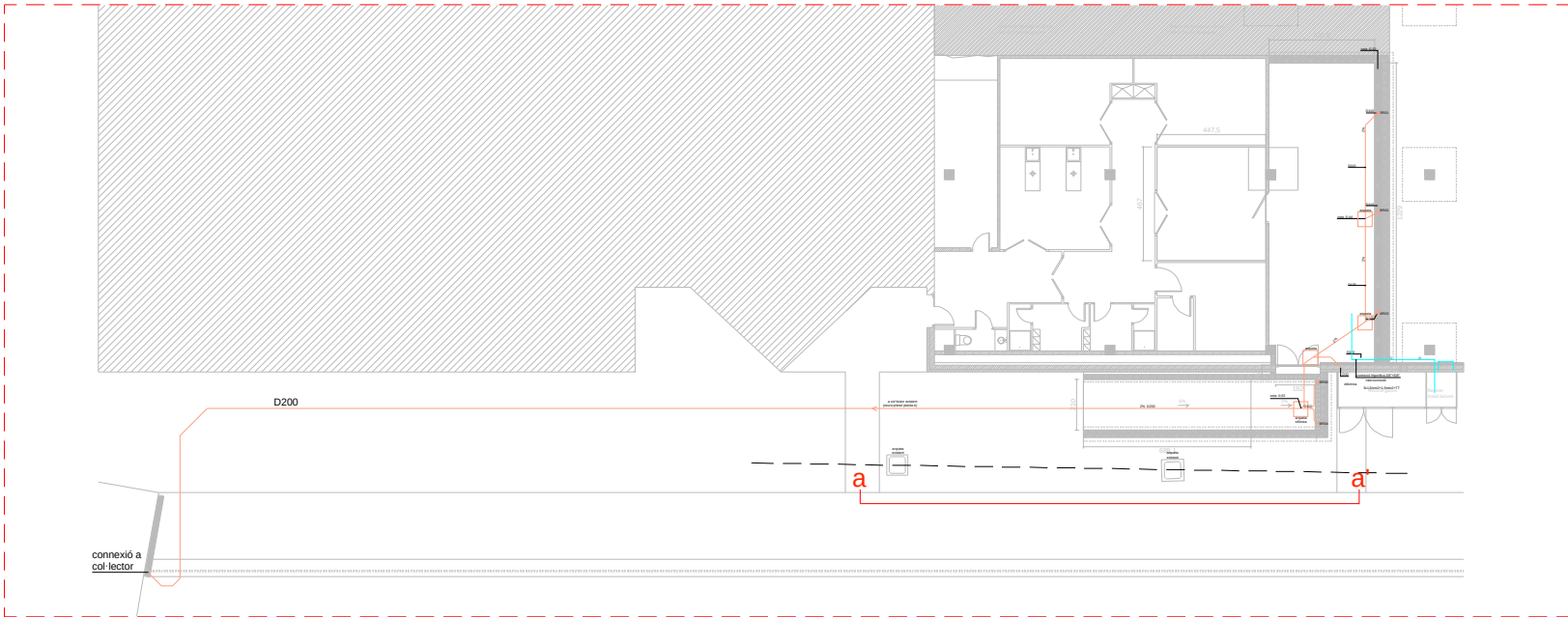
Planta A e: 1/300 Connexió a col·lector existent
