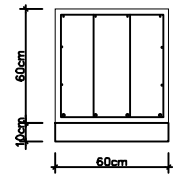
SABATA 60x60 60x60 arm. superior 4ø16, arm. inferior 4ø20, 4ø12 de pell, 1ø4Rø8c/25. 10cm de formigó de neteja
