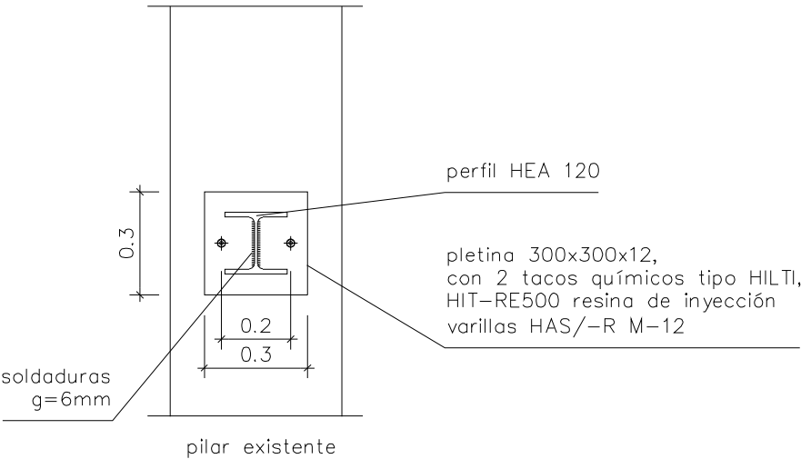
ENTREGA TIPO 2 ESCALA 1/2o
