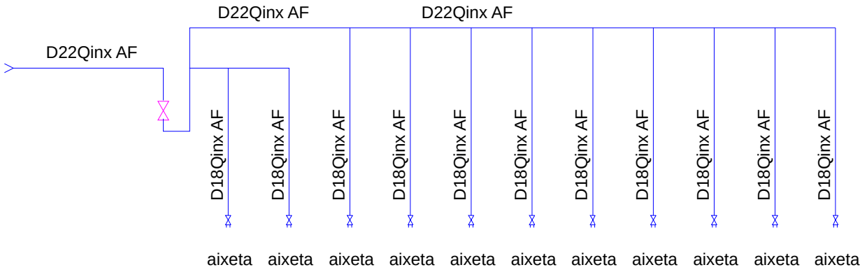
Esquema aigua potable
