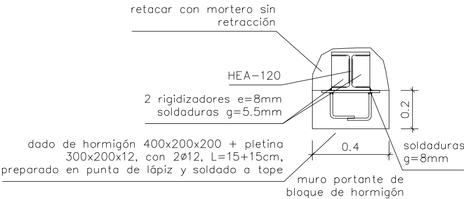
ENTREGA TIPO 1 ESCALA 1/2o
