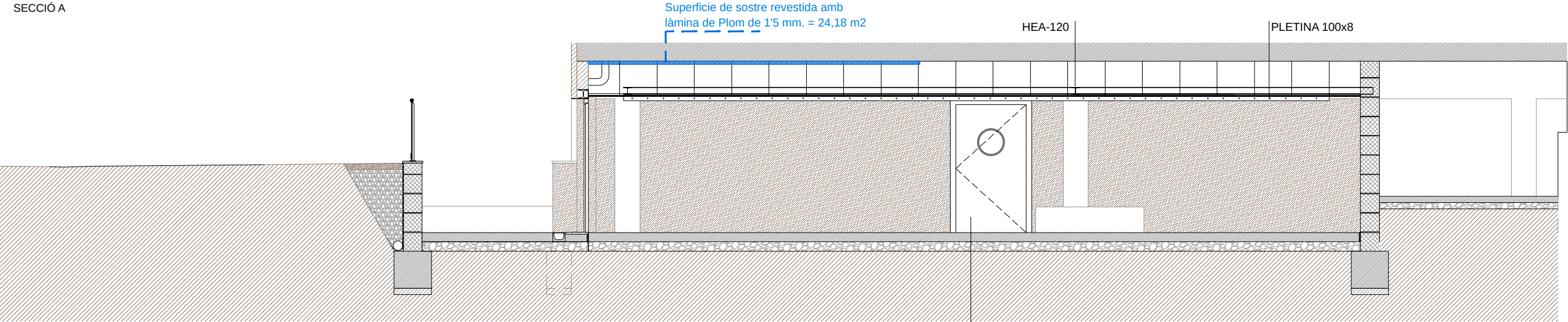
SECCIÓ B
