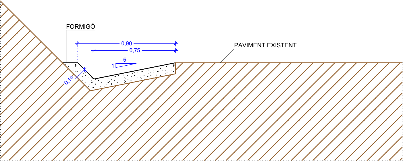
DETALL CUNETA AMERICANA
