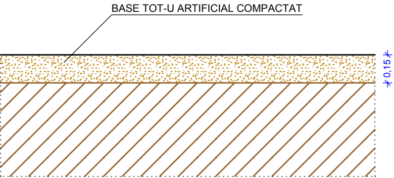
SECCIÓ TRANSVERSAL - MILLORA DEL FERM
