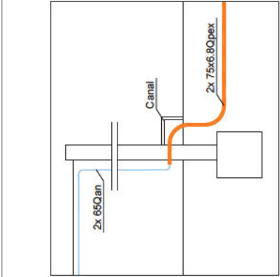
Detall entrada circuit hidràulic vestuaris pavelló E. 1/50
