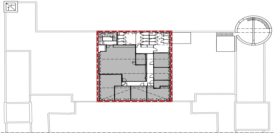
PLANTA TERCERA
