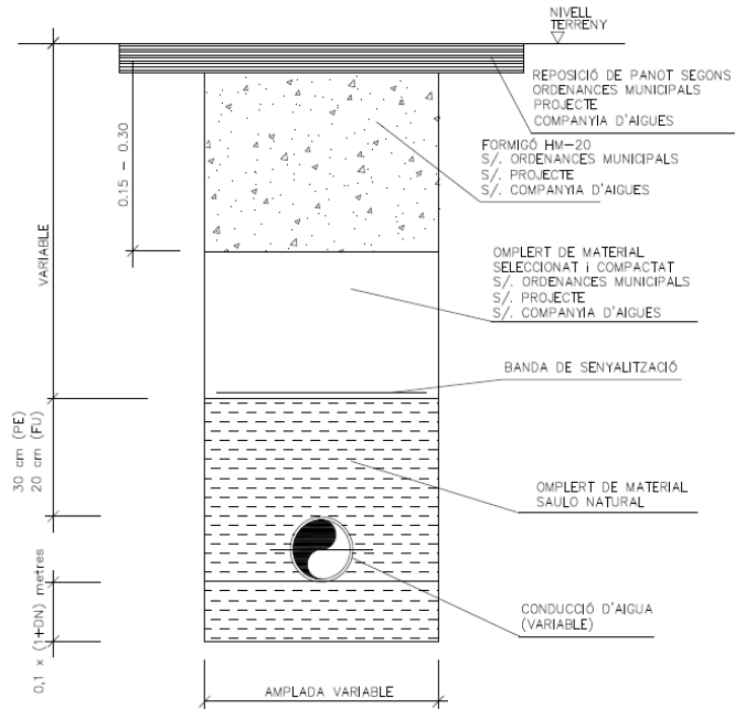
SECCIÓ TIPUS RASA CONDUCCIÓ AIGUA EN VORERA
