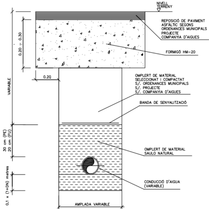
SECCIÓ TIPUS RASA CONDUCCIÓ AIGUA EN CALÇADA
