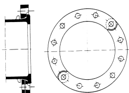
Brida orientable
