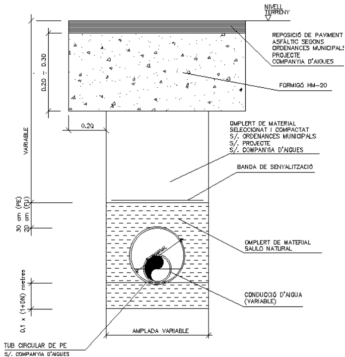
SECCIÓ TIPUS RASA CONDUCCIÓ AIGUA EN CALÇADA
