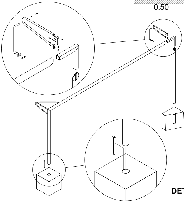
DETALL MUNTATGE ESCAIRE
