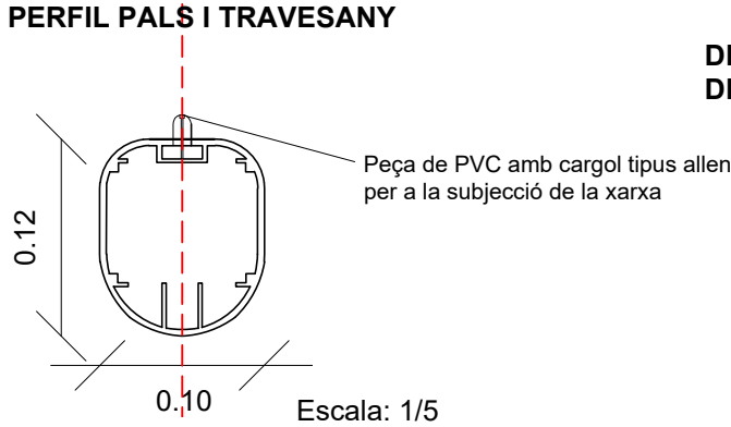
DETALL PERFIL PALS I TRAVESANY
