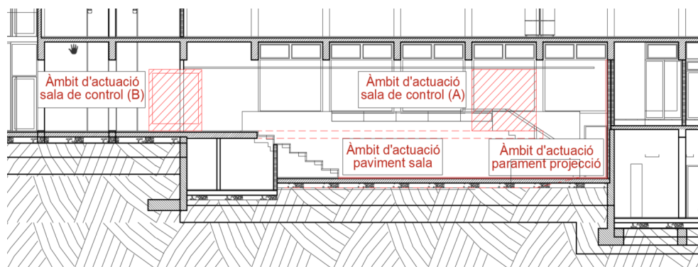
Fig.4: Àmbits d'actuació en secció
