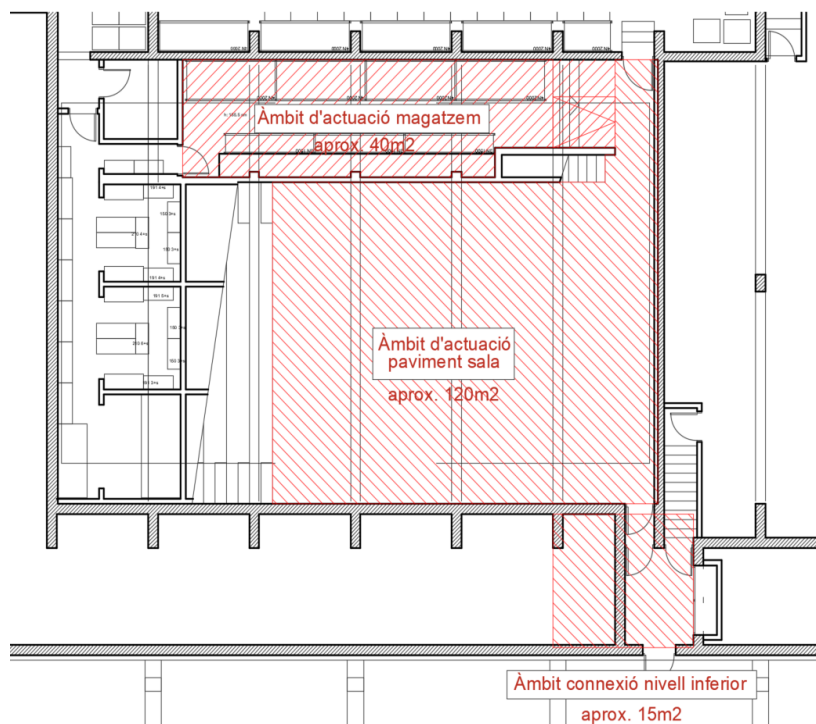
Fig.3: Planta Nivell inferior: àmbit d'actuació paviment nivell inferior, àmbit de magatzem i àmbit de connexió nivell inferior
