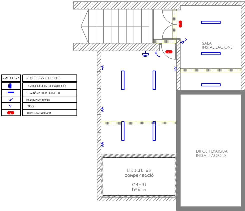
PLANTA RECEPTORS ELÈCTRICS INSTAL·LACIONS
