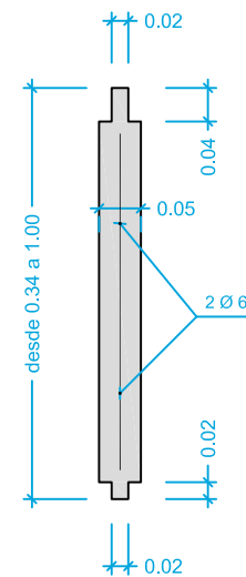
Planta
