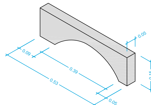
Cornisa lateral dreta
