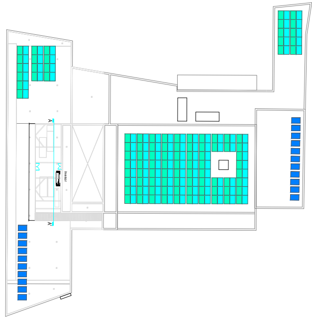
Planta Auditori E: 1/750
