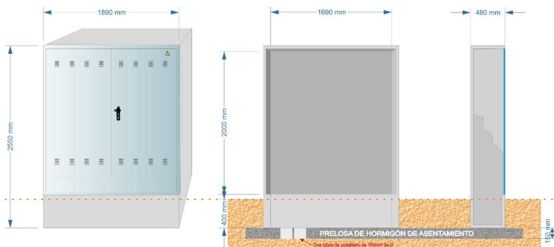
Dimensions de l'armari prefabricat monobloc
