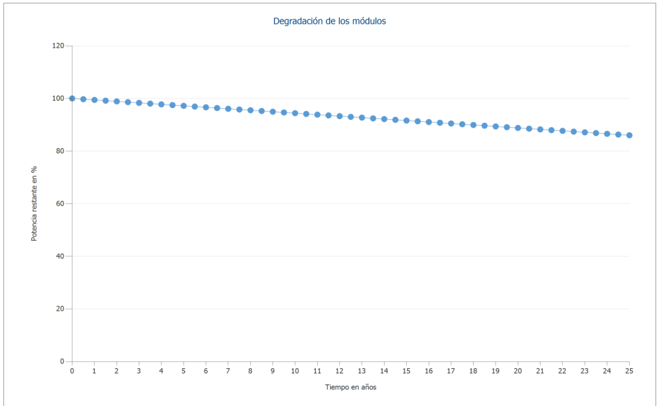
Figura: Degradación de los módulos, 1. Superficie fotovoltaica - Edificio a discreción 04-Superficie a ocupar Oeste
