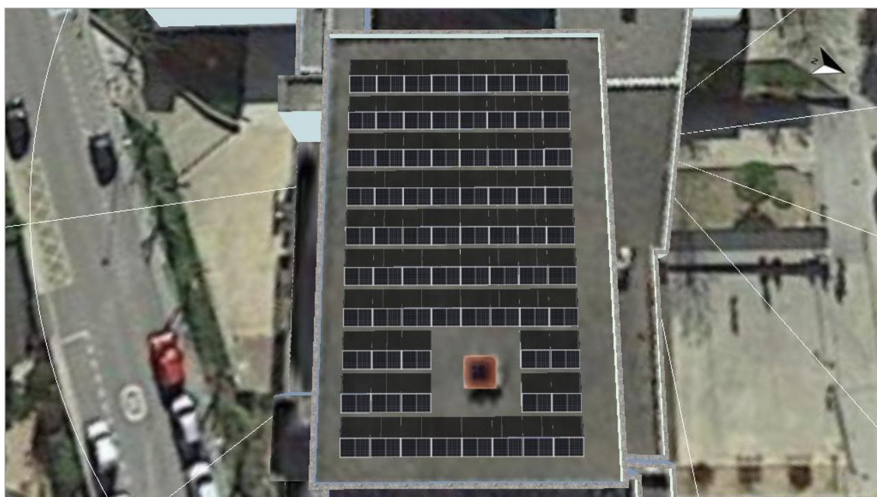
Figura: 8. Superficie fotovoltaica - Edificio 01-Superficie fotovoltaica Este
