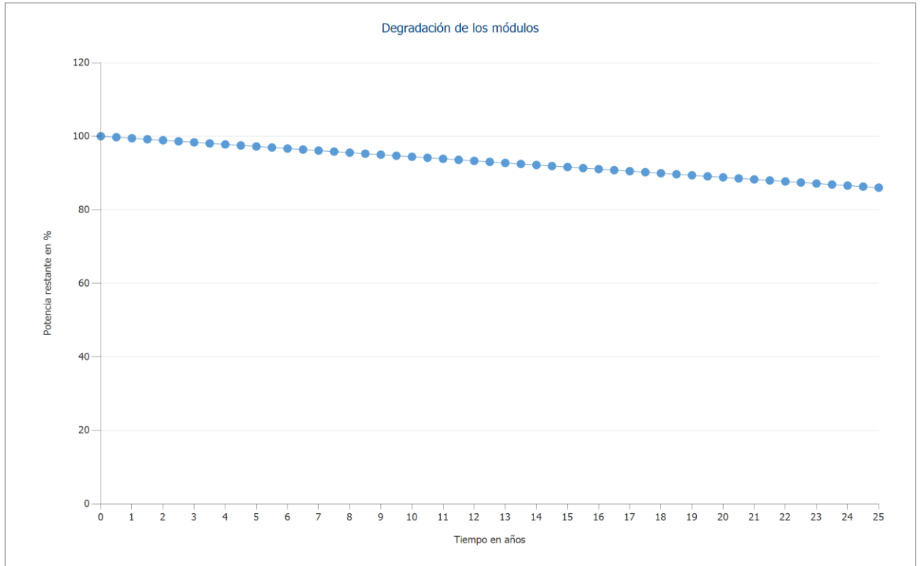
Figura: Degradación de los módulos, 6. Superficie fotovoltaica - Edificio a discreción 03-Superficie fotovoltaica Este
