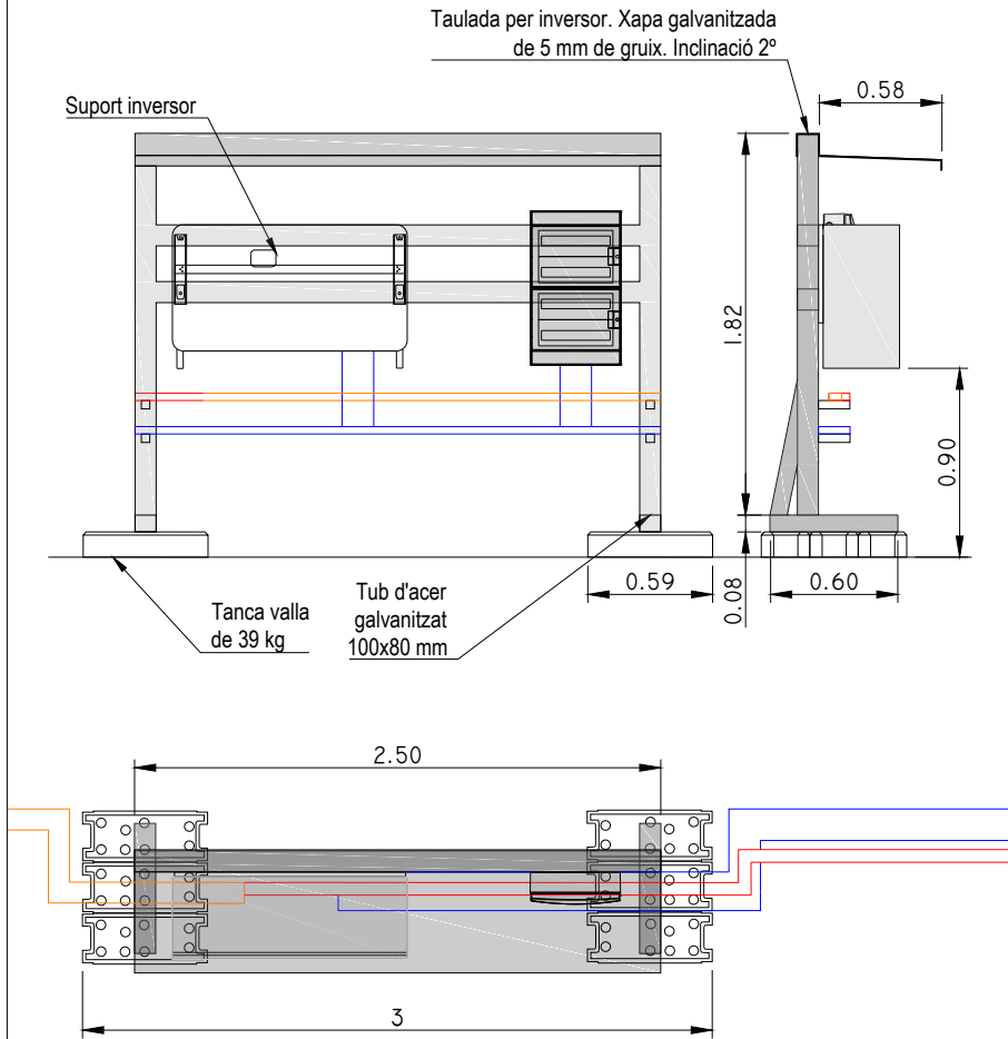
Detall Estructura Inversor E: 1/40
