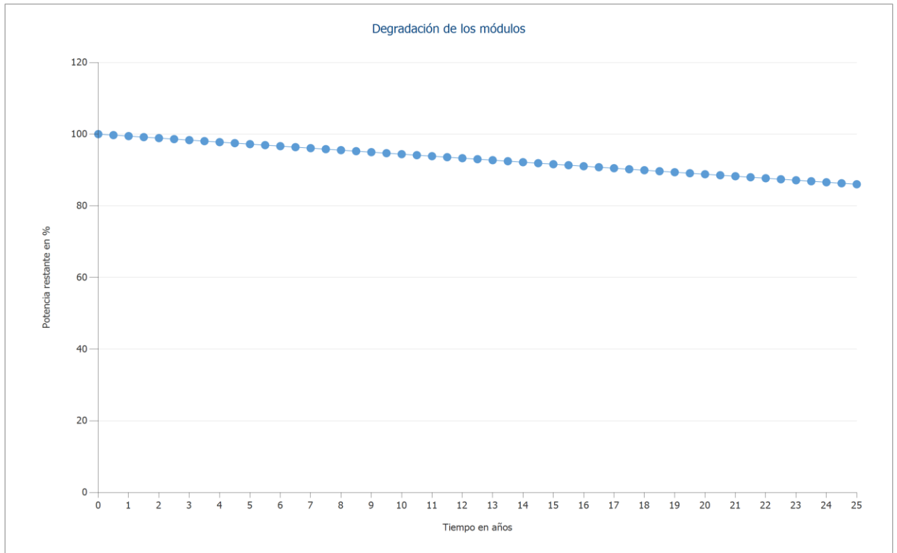
Figura: Degradación de los módulos, 4. Superficie fotovoltaica - Edificio a discreción 04-Superficie fotovoltaica Nordeste
