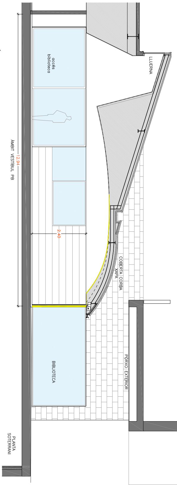
SECCIÓ SL-2 SECCIÓ LONGITUDINAL-2 PER ACCÉS 0m 1m 2m 3m 4m ESCALA GRÀFICA 1/100
