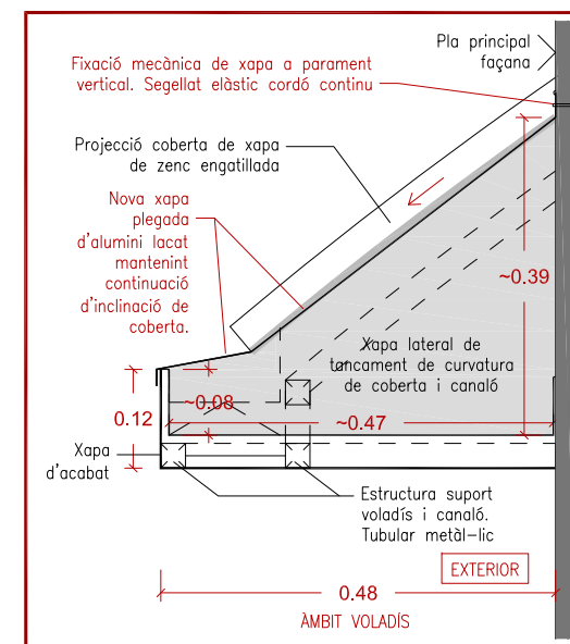
PROPOSTA, DETALL -A- SECCIÓ DETALL -A- CONTINUACIÓ DE COBERTA CORBA
