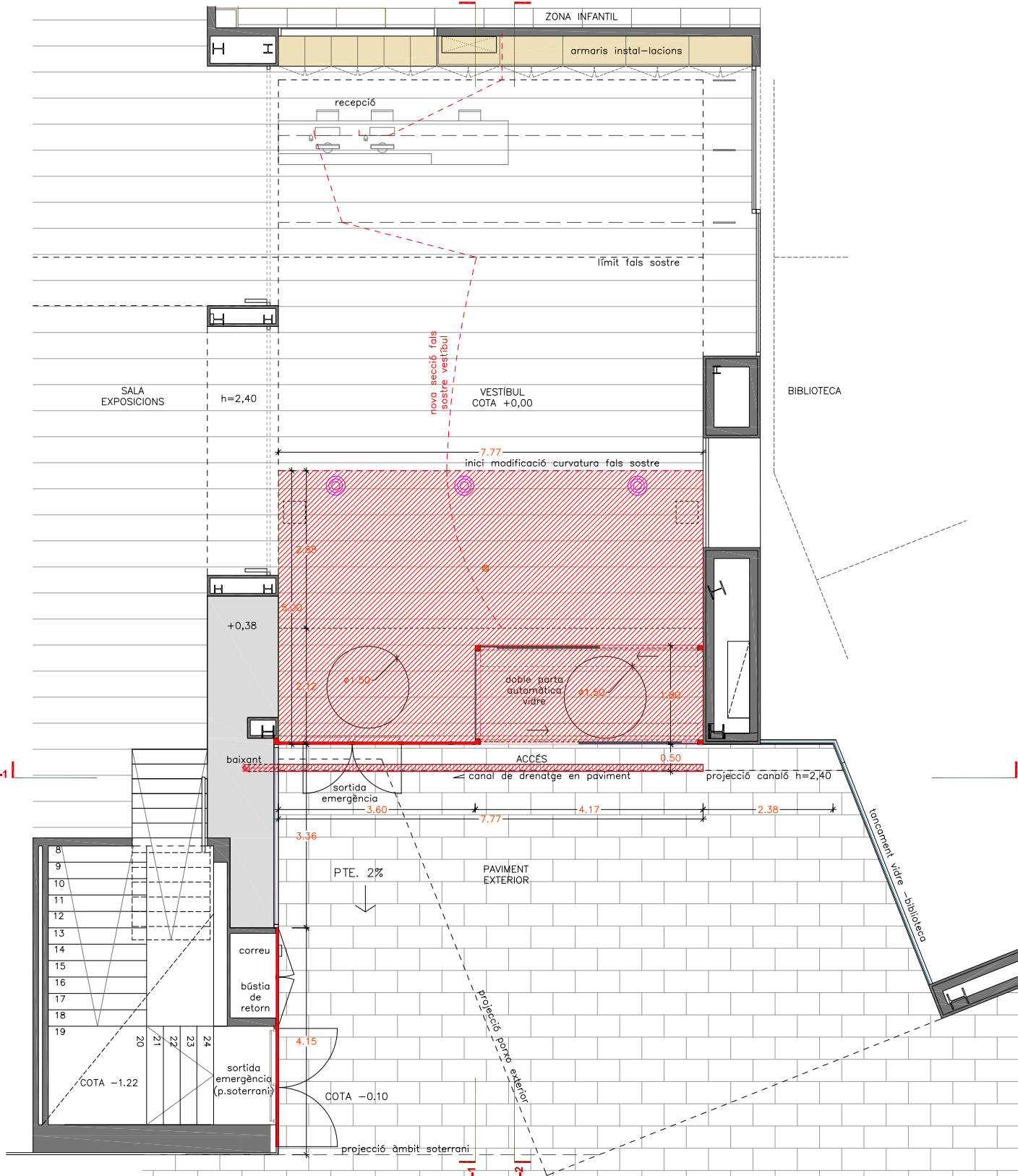
PLANTA PLANTA BAIXA ACCÉS CENTRE CÍVIC ATENEU 0m 1m 2m 3m 4m ESCALA GRAFICA 1/100
