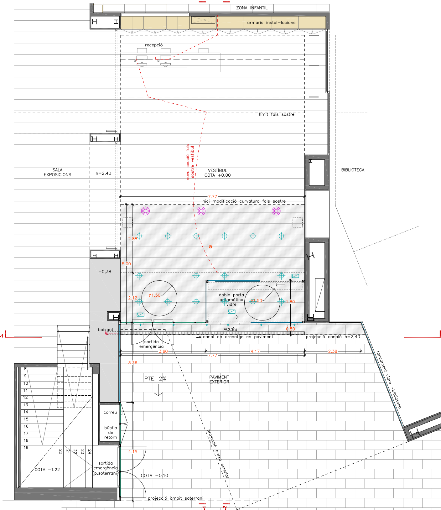
PLANTA PLANTA BAIXA ACCÉS CENTRE CÍVIC ATENEU 0m 1m 2m 3m 4m ESCALA GRÀFICA 1/100
