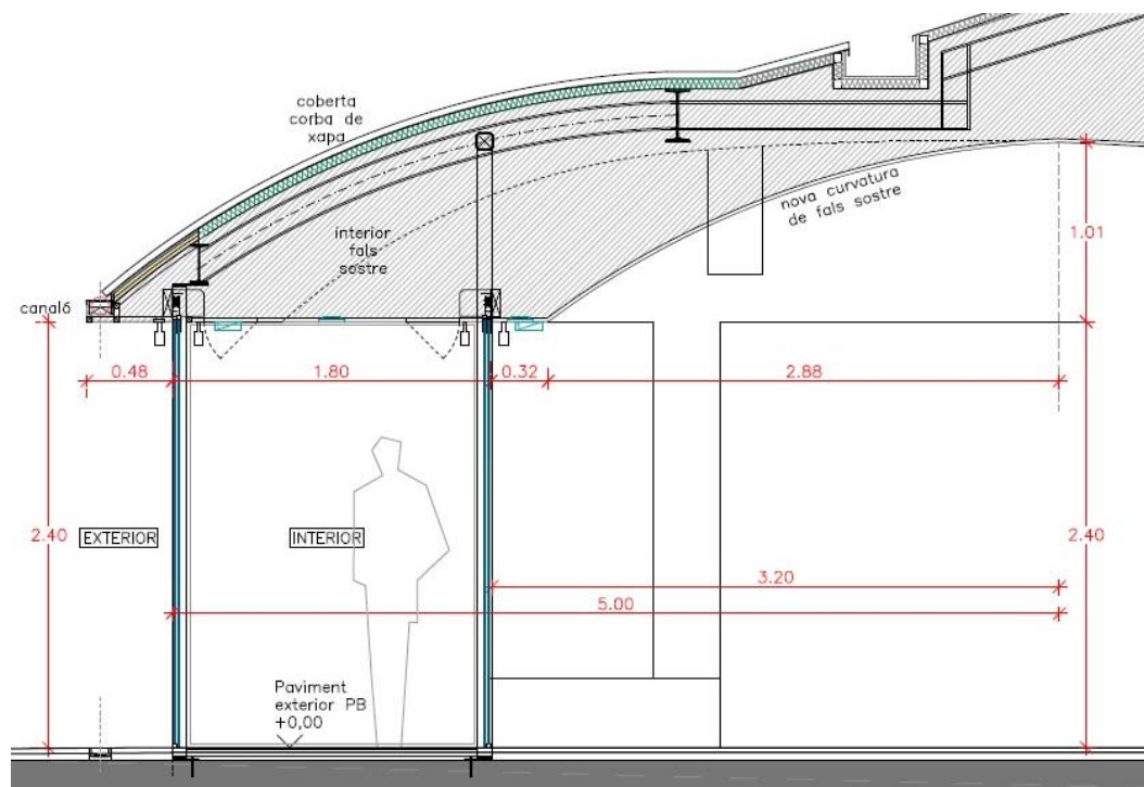
Plànol. Planta i alçat de fusteria frontal. Doble porta i àmbit de nova curvatura de fals sostre.
