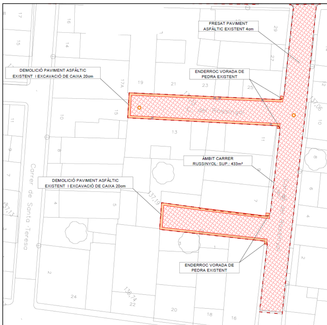
Figura 26. Demolicions i enderrocs del carrer Russinyol.
