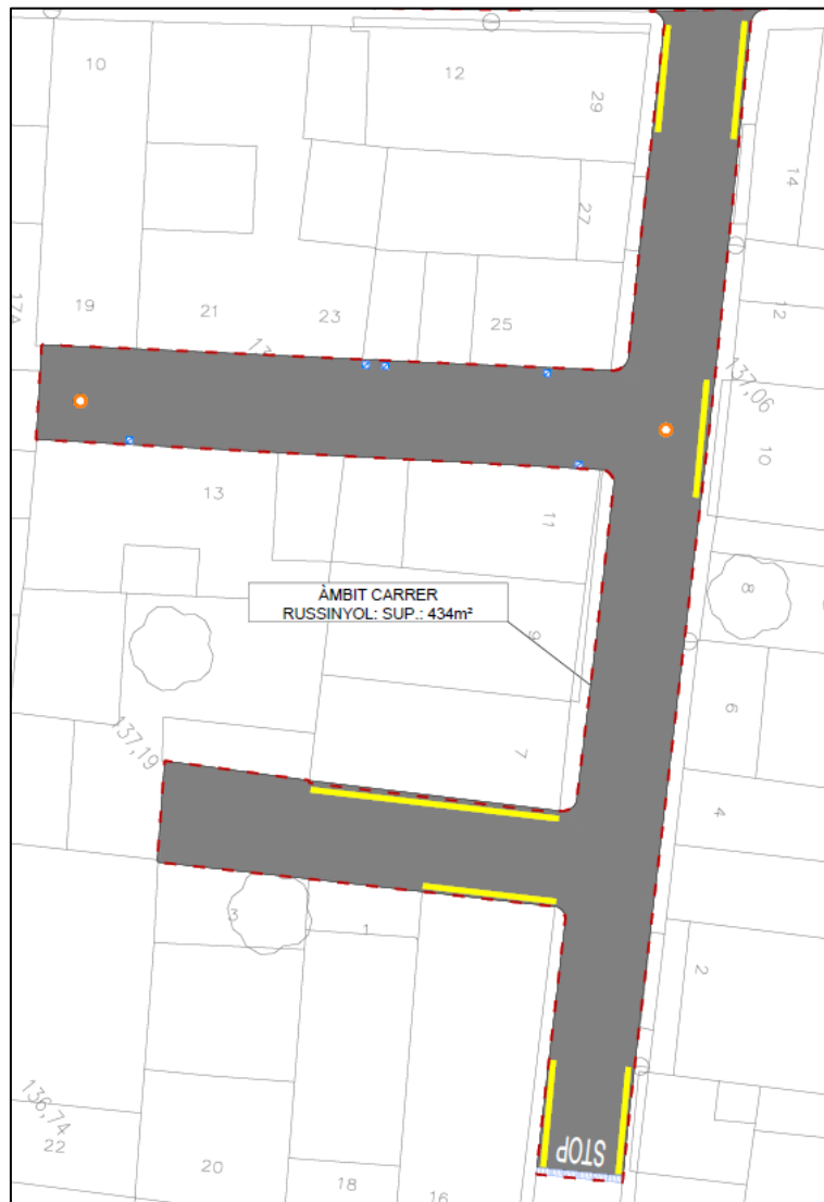
Figura 8. Estat actual del carrer Russinyol.
