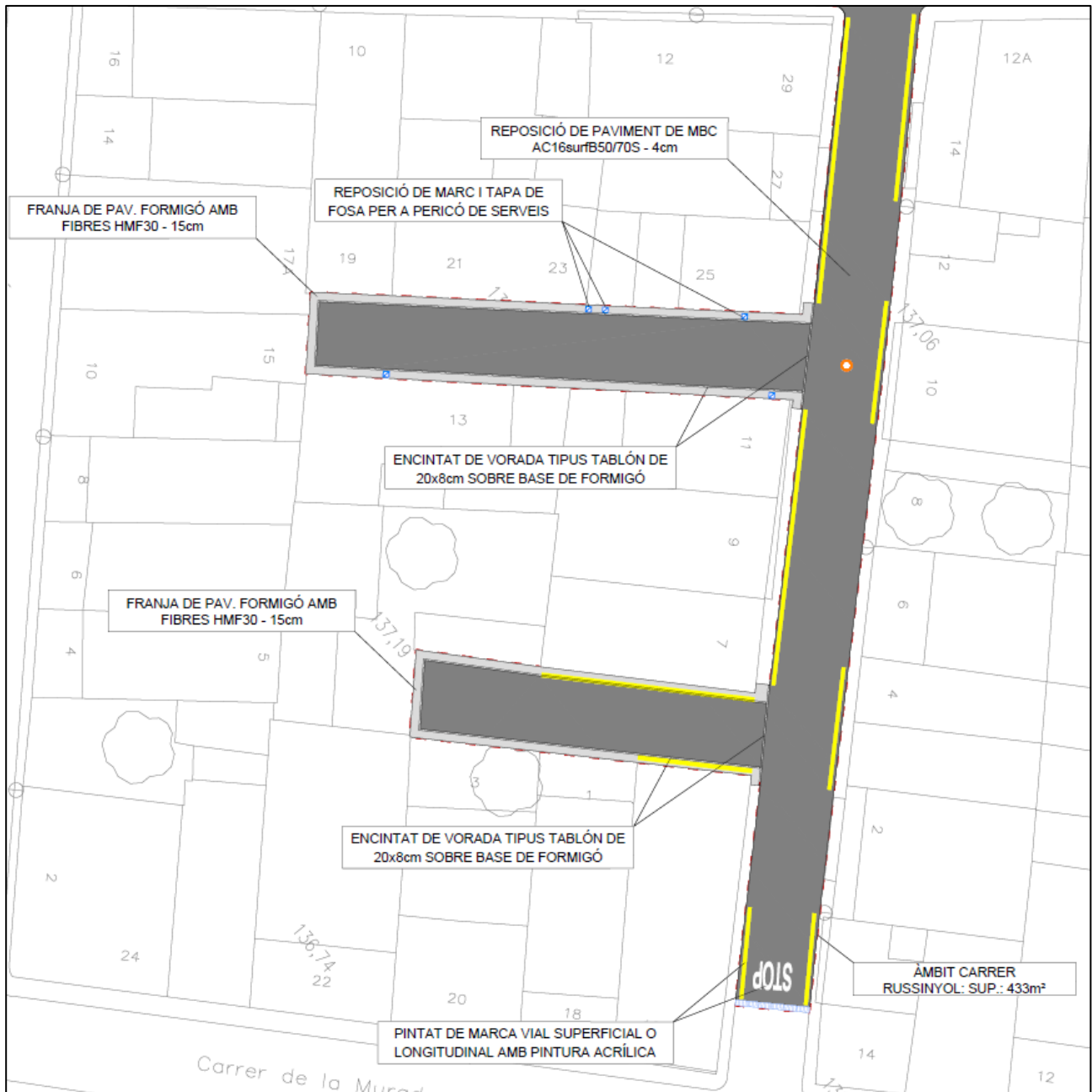
Figura 5. Carrer Russinyol amb els dos carrerons transversals.
