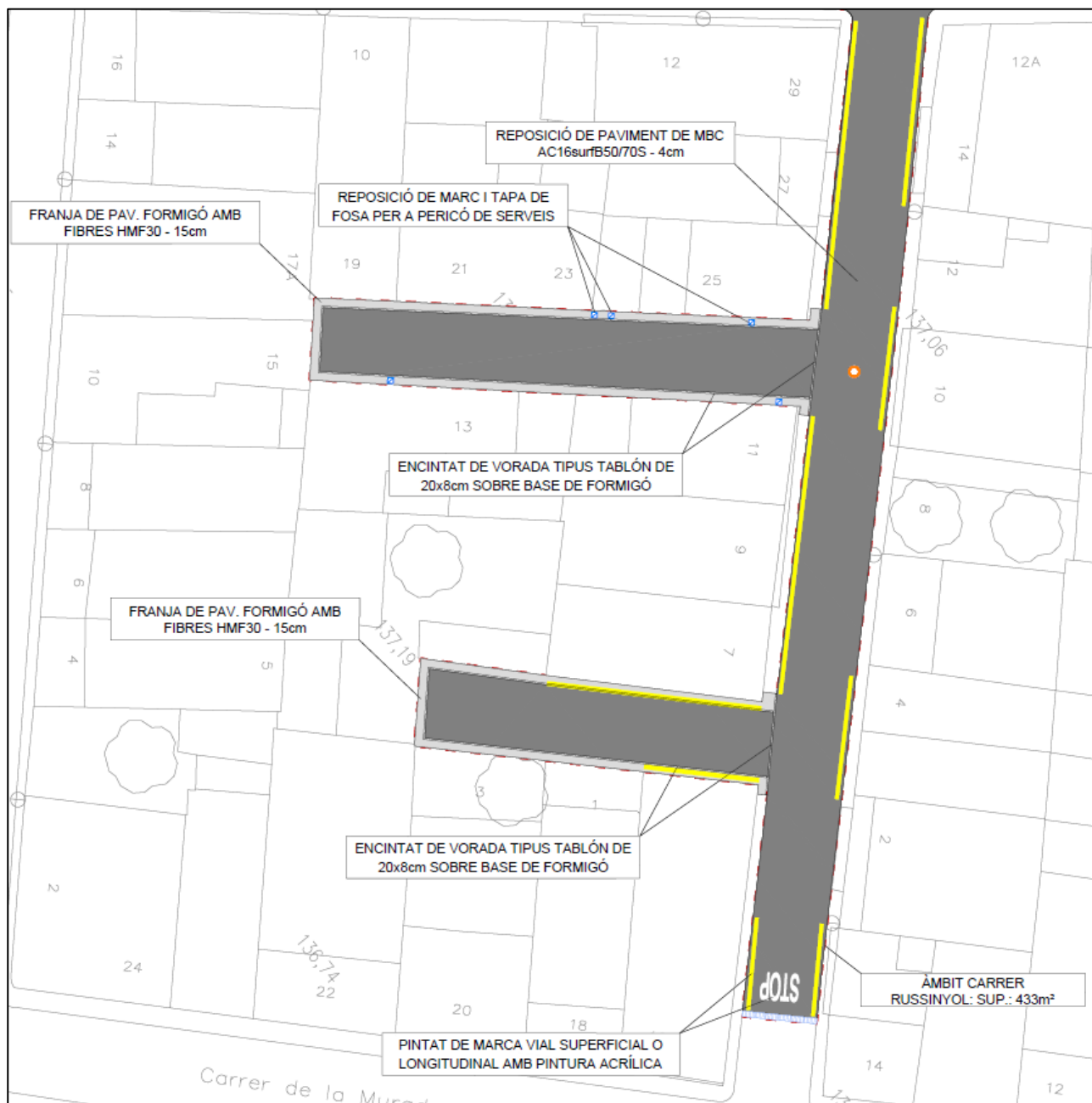
Figura 31. Carrer Russinyol amb els dos carrerons transversals.
