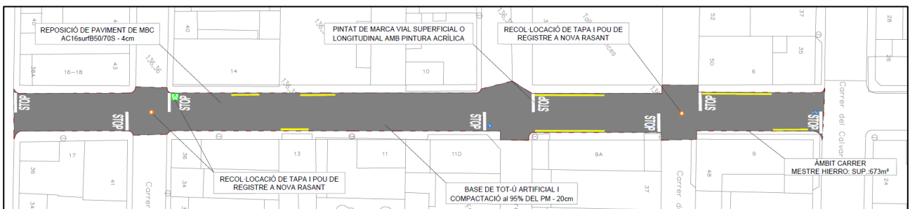
Figura 28. Carrer Mestre Hierro.
