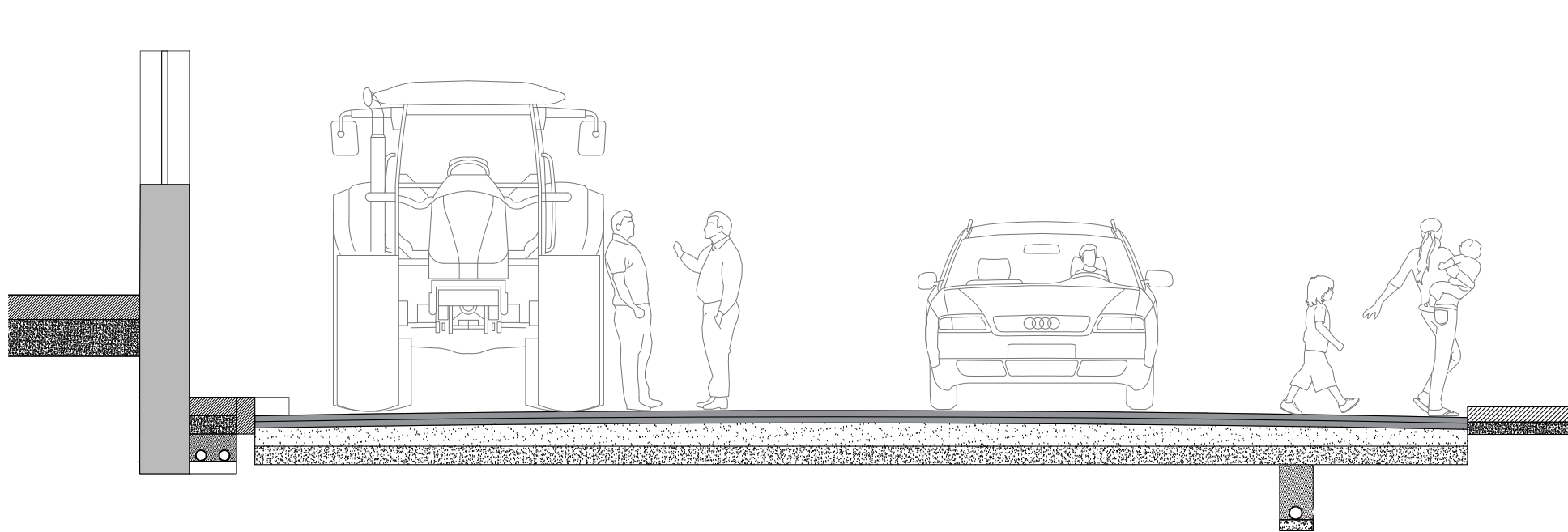
secció A-A' estat actual 0.54 9.90 0.85
