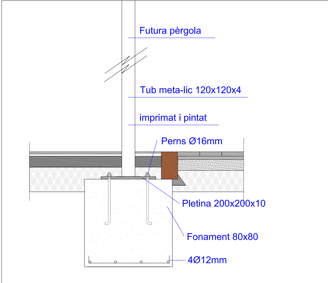
DETALL 4 fonament estructura futura marquesina
