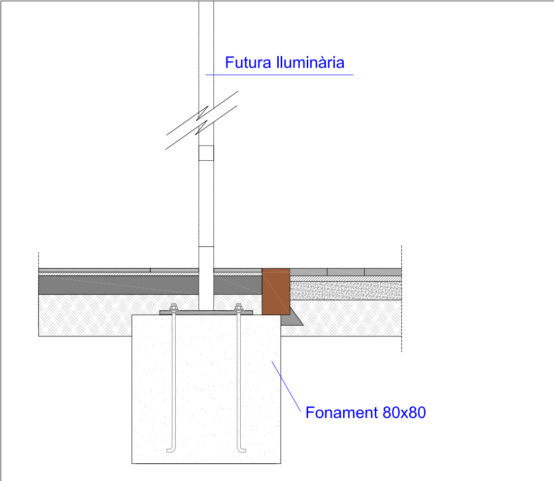
DETALL 3 fonament fanal
