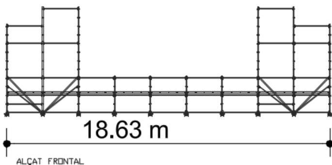
ALÇAT FRONTAL
