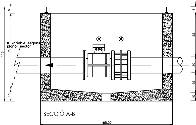
ARQUETA COMPTADOR (95 x 165 cm)
