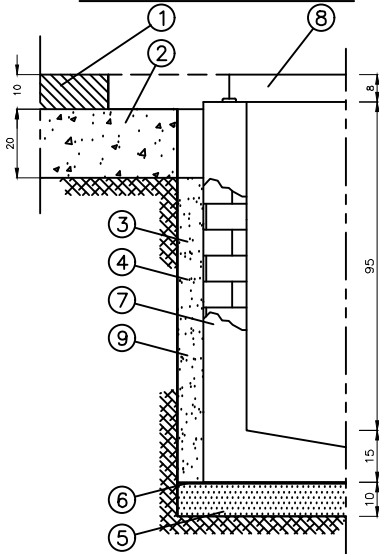
DETALL SECCIÓ ARQUETA
