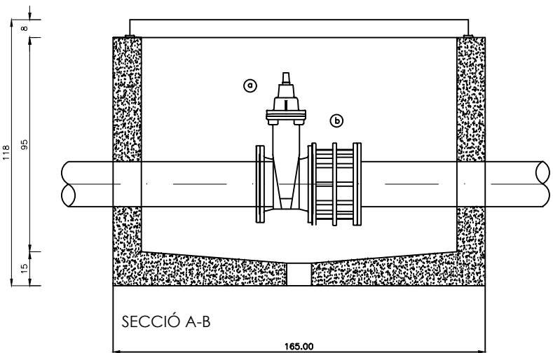
ARQUETA VÀLVULA (95 x 165 cm)
