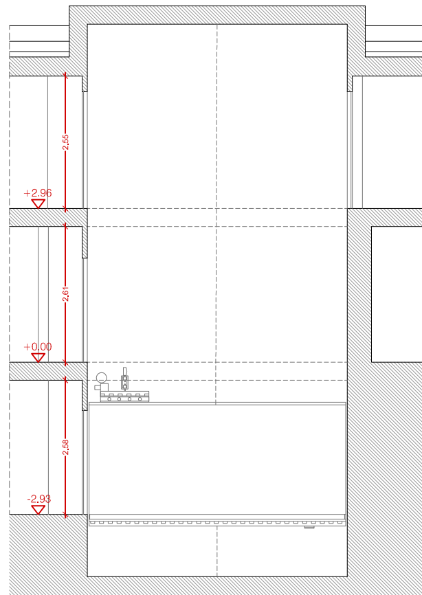
SECCIÓ A-A'
