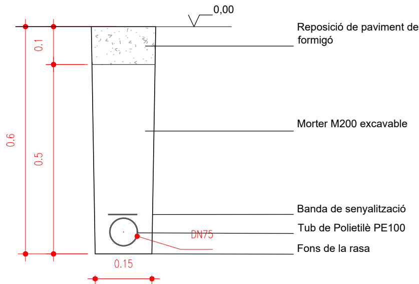
SECCIÓ RASA 15 CM PER TUB DE DN75
