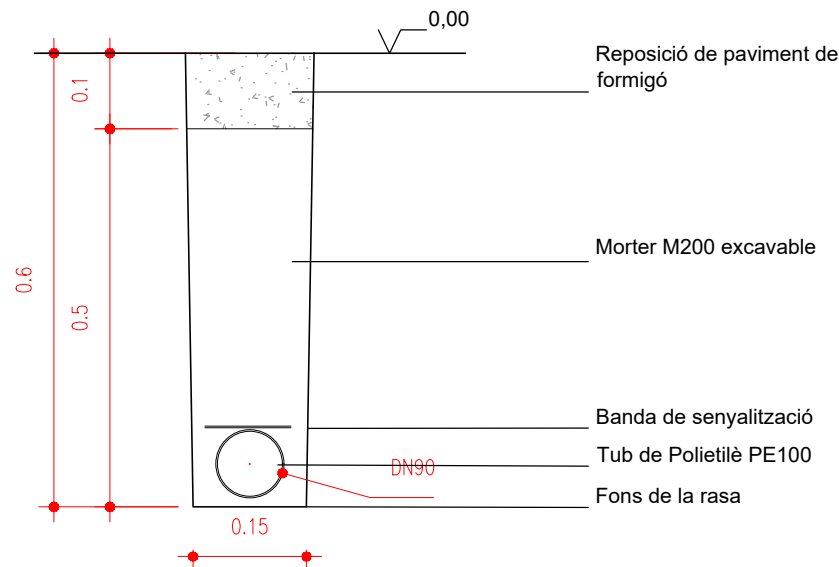
SECCIÓ RASA 15 CM PER TUB DE DN90
