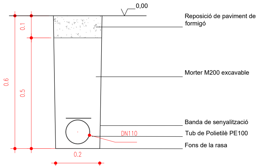
SECCIÓ RASA 20 CM PER TUB DE DN110
