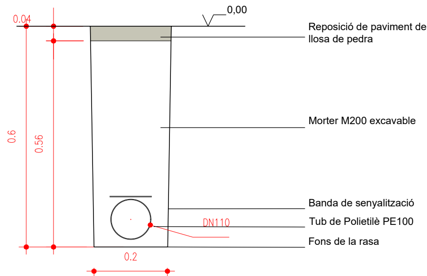
SECCIÓ RASA 20 CM PER TUB DE DN110 ACABAT AMB LLOSA DE PEDRA
