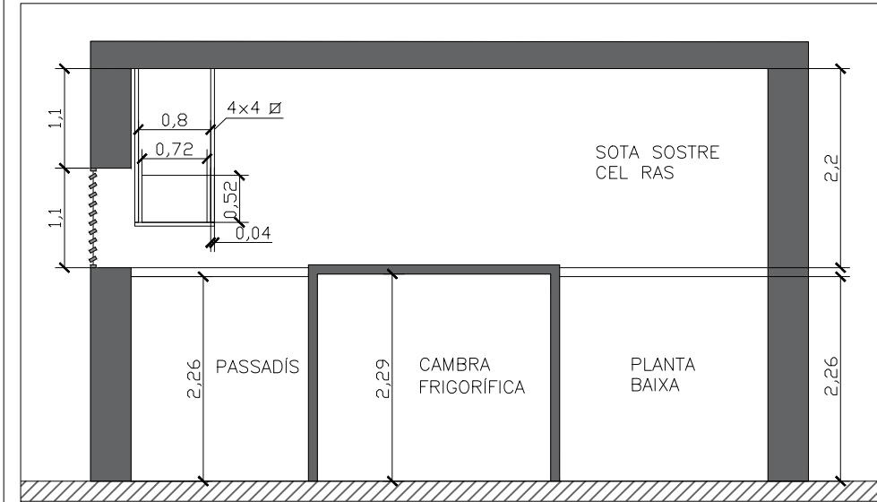
SECCIÓ A-A'
