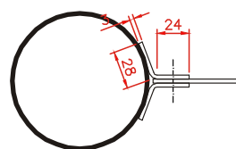
Detall forat passant
