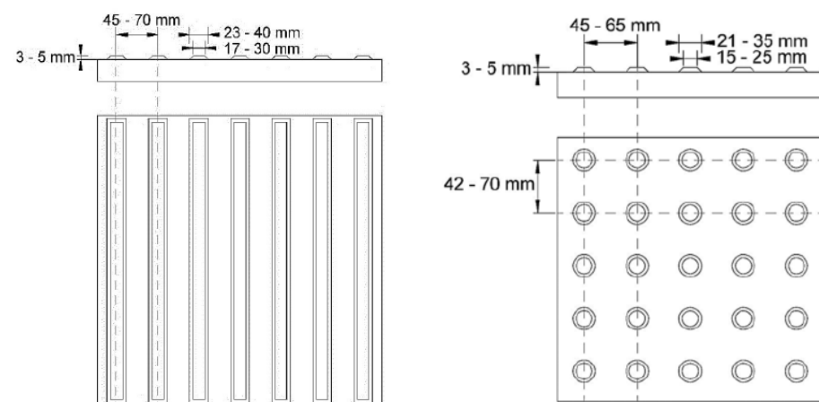
Figura 14. Característiques específiques dels paviment podotàcil segons el Codi d'Accessibilitat
