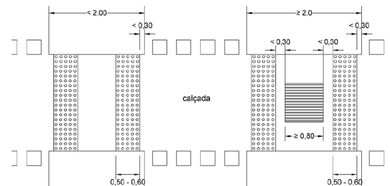
Figura 2a.9. Exemples de pavimentació tàtil en illot intermedi
