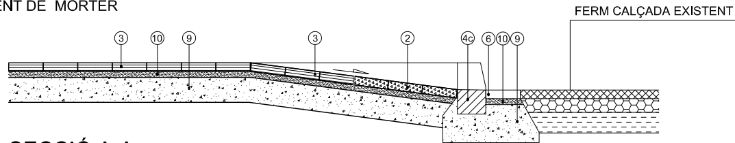
SECCIÓ A-A
