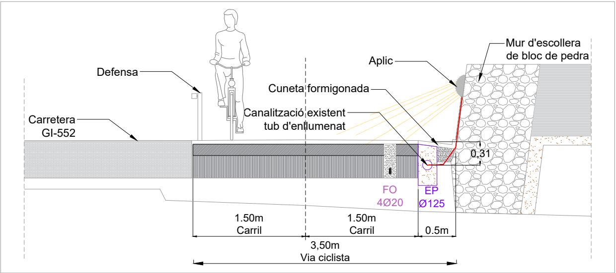
S1 - DETALL SECCIÓ MUR APLIC 1/50
