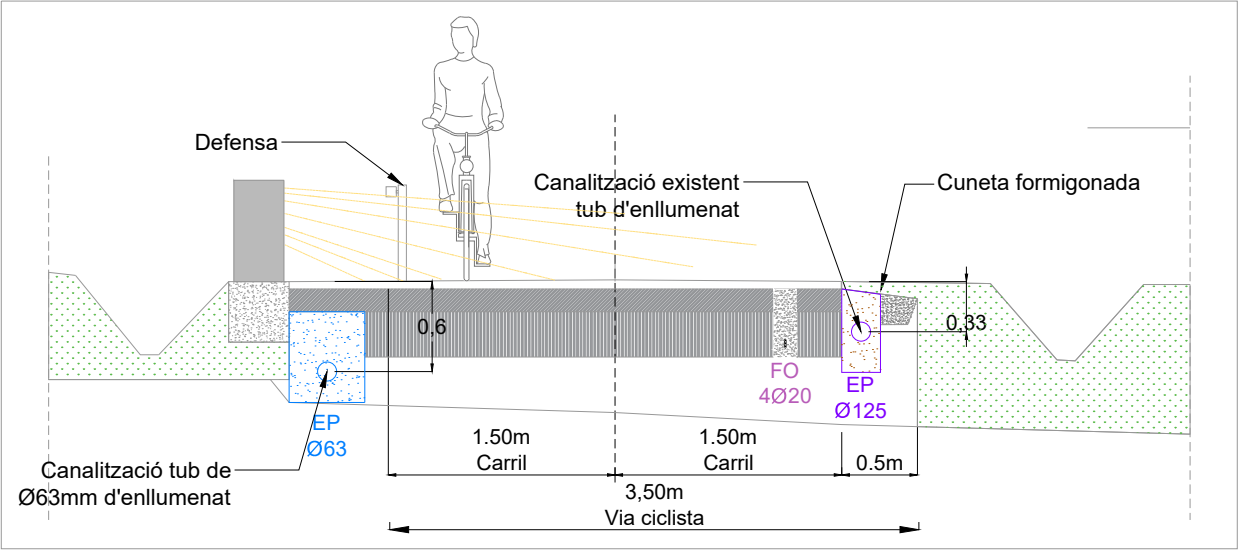
S3 - DETALL SECCIÓ BALISA TRAM BREDÀ CANVI DE COSTAT 1/50
