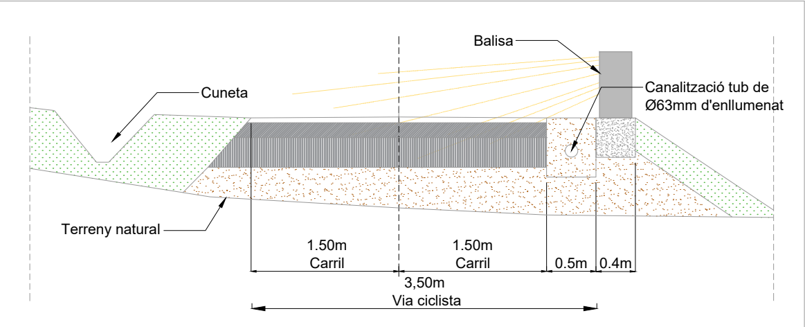
SECCIÓ TIPUS BALISA 1/100
