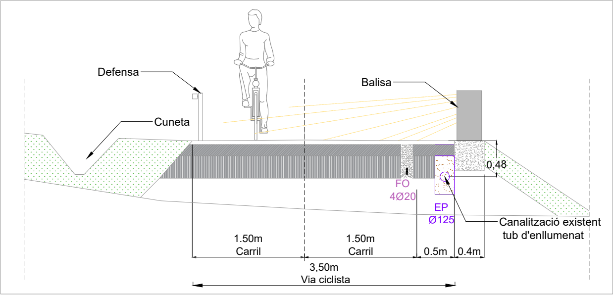
S2 - DETALL SECCIÓ BALISA TRAM BREDÀ 1/50
