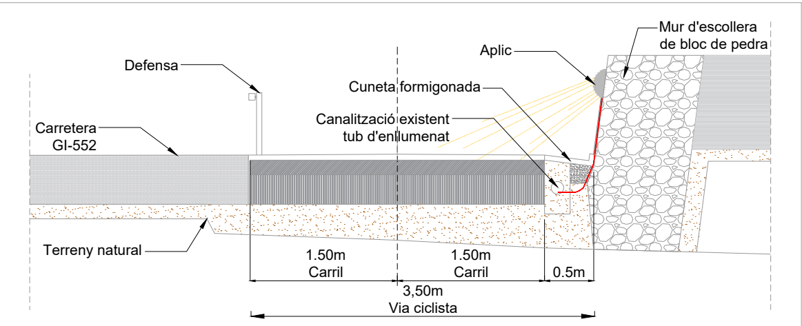
SECCIÓ TIPUS APLIC MUR 1/100
