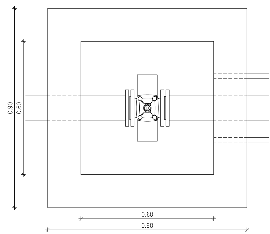
PLANTA
