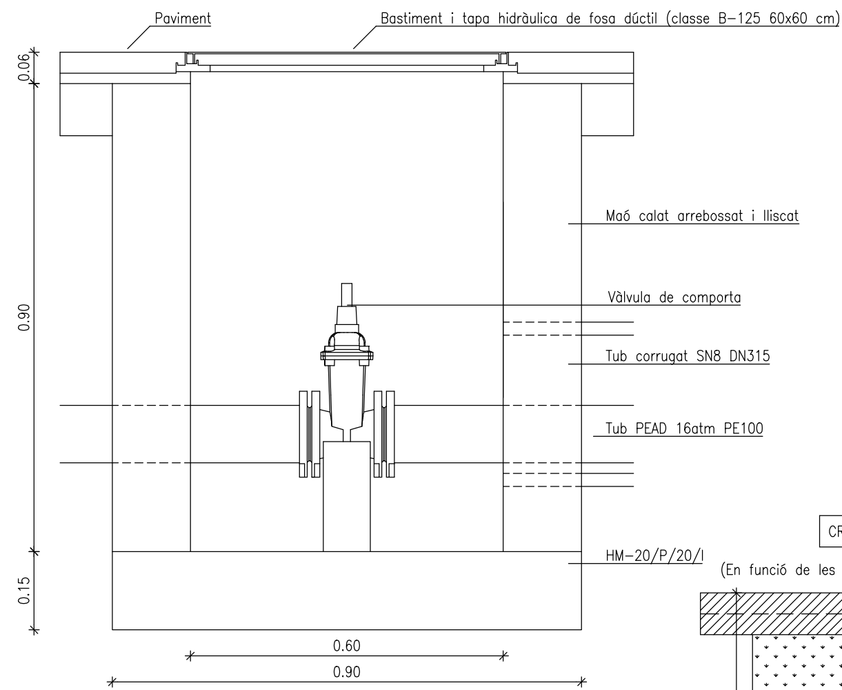
SECCIÓ
