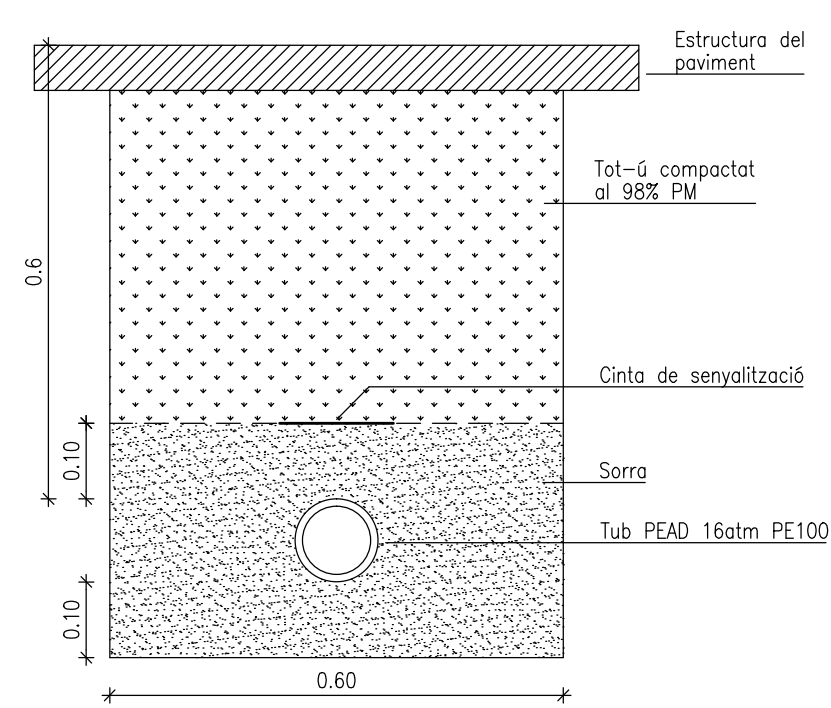
CREUAMENT CARRETERA
