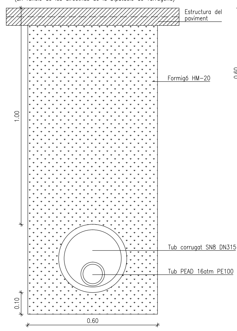
CREUAMENT CARRETERA
