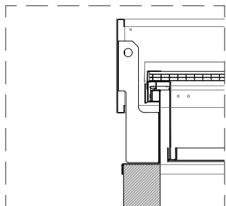
DETALLE 01 aluminio simple
