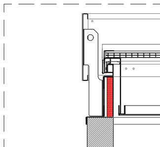
DETALLE 02 aluminio doble con aislamiento
