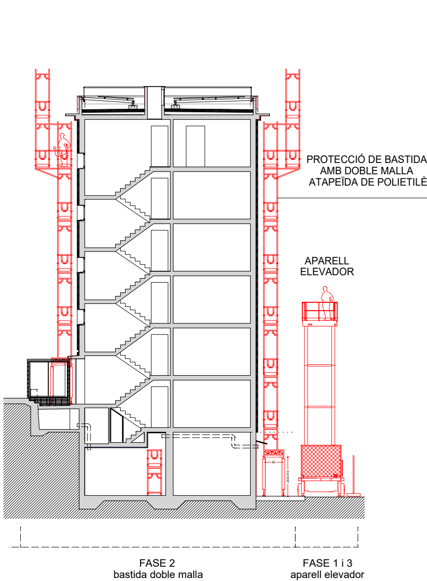
SECCIÓ E. 1:200
