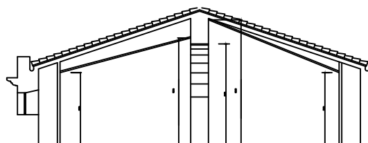
SECCIO TRANSVERSAL
