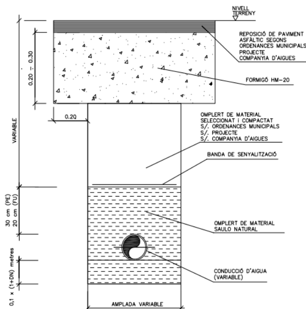
SECCIÓ TIPUS RASA CONDUCCIÓ AIGUA EN CALÇADA
