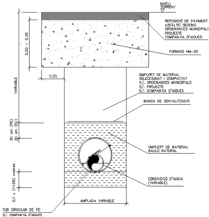
SECCIÓ TIPUS RASA CONDUCCIÓ AIGUA EN CALCADA
