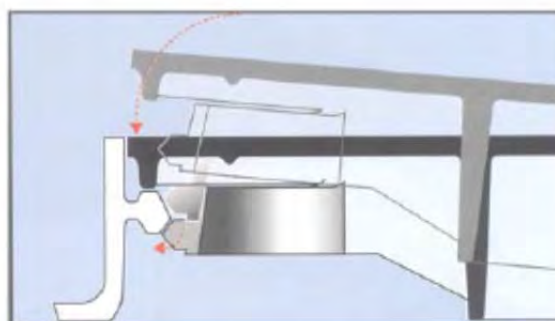
DETALL BLOQUEIG
