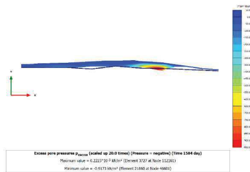
Figura 3.4.6. Fase llarg termini (Consolidació a llarg termini, 95%). Excés de pressions de porus. Secció BB'.
