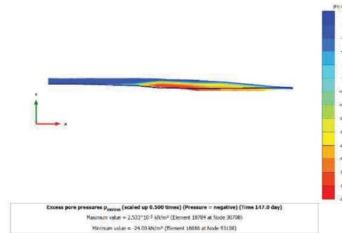
Figura 3.4.7. Fase intermèdia (Col·locació graves drenants). Excés de pressions de porus. Secció CC'.
