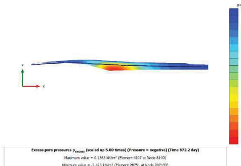
Figura 3.1.6. Fase llarg termini (Consolidació a llarg termini, 95%). Excés de pressions de porus. Secció AA'.
