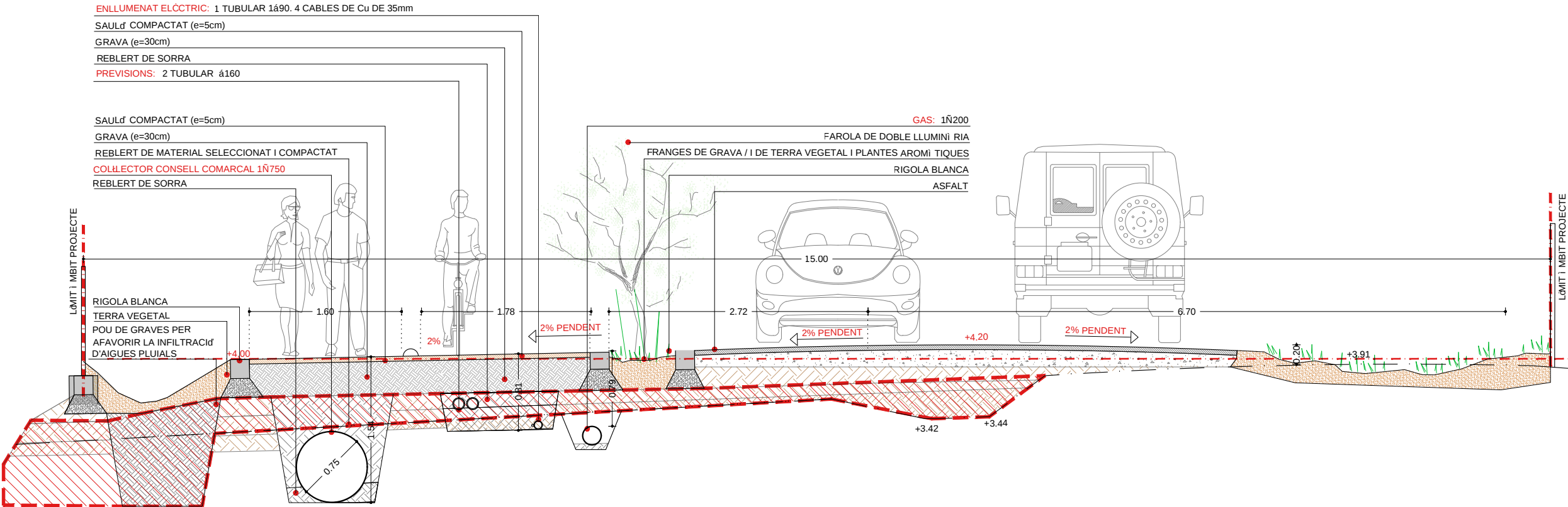
SECCIó 9. E:1/50
