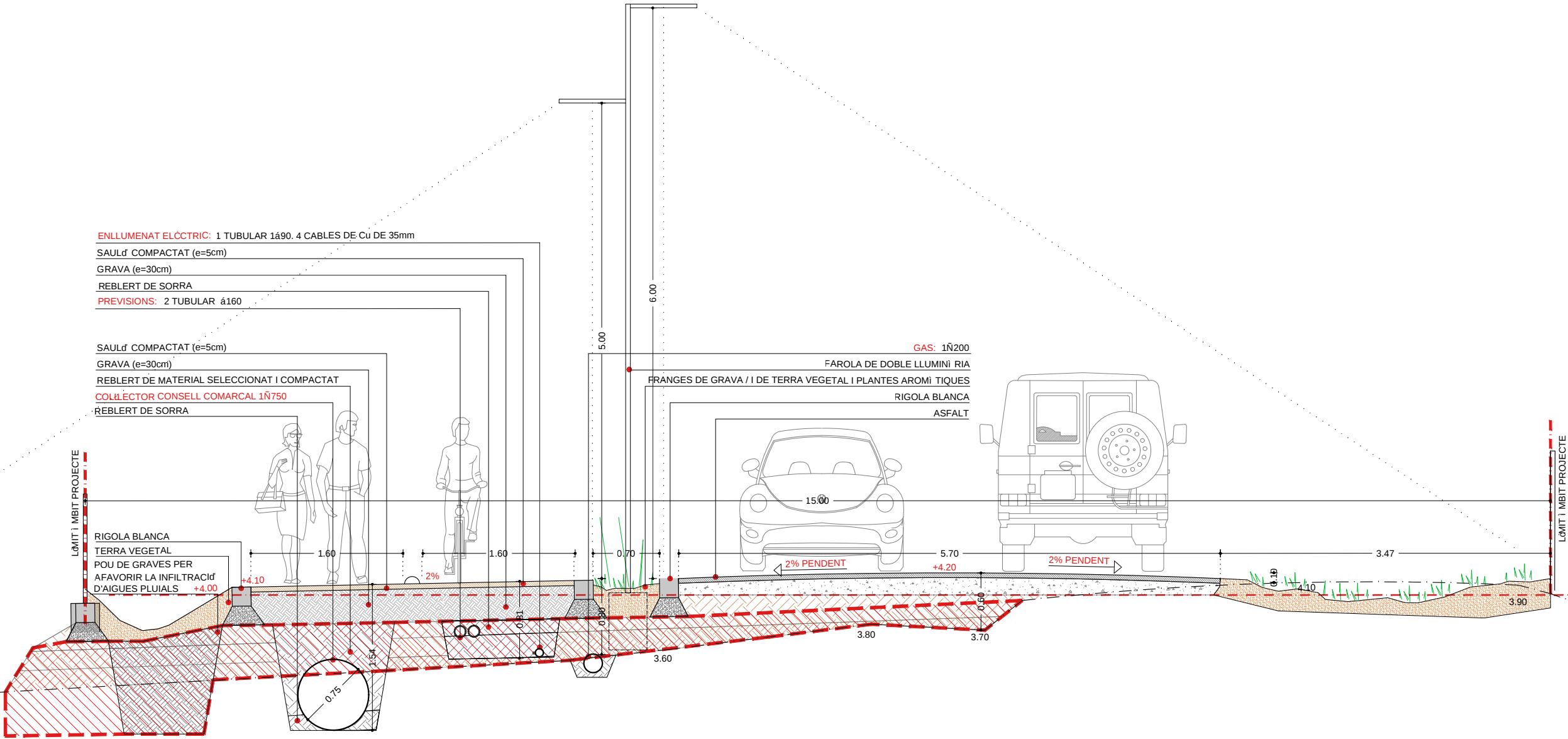
SECCIÓ 3. E:1/50
