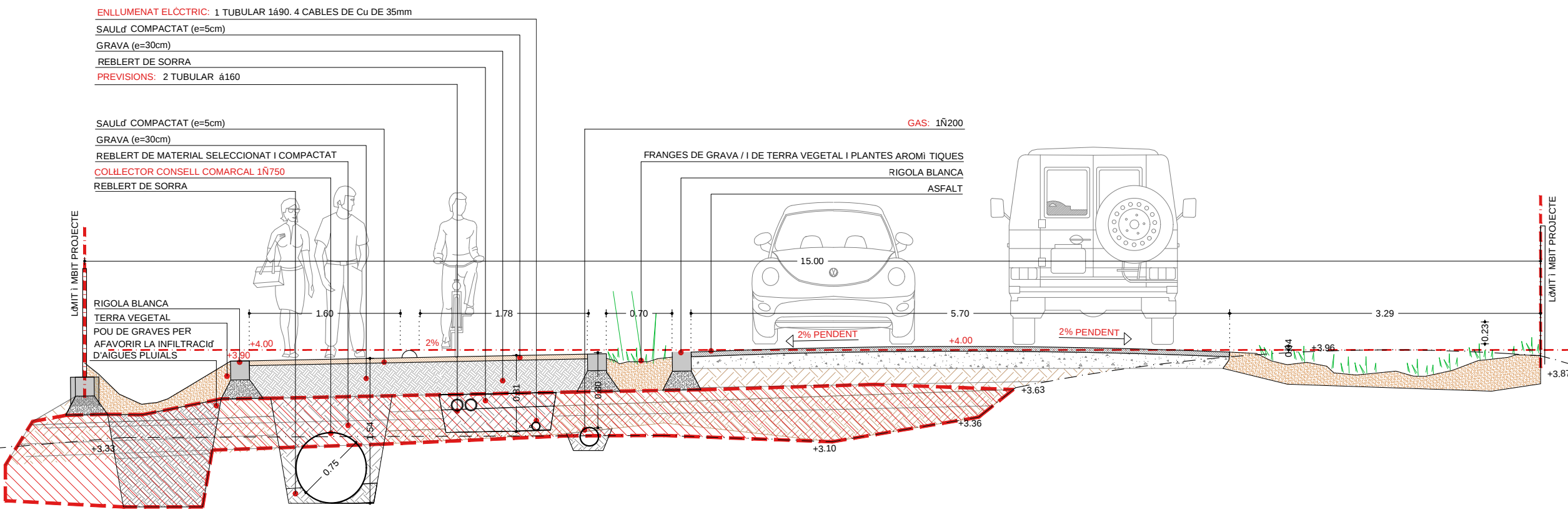
SECCIÓ 5. E:1/50
