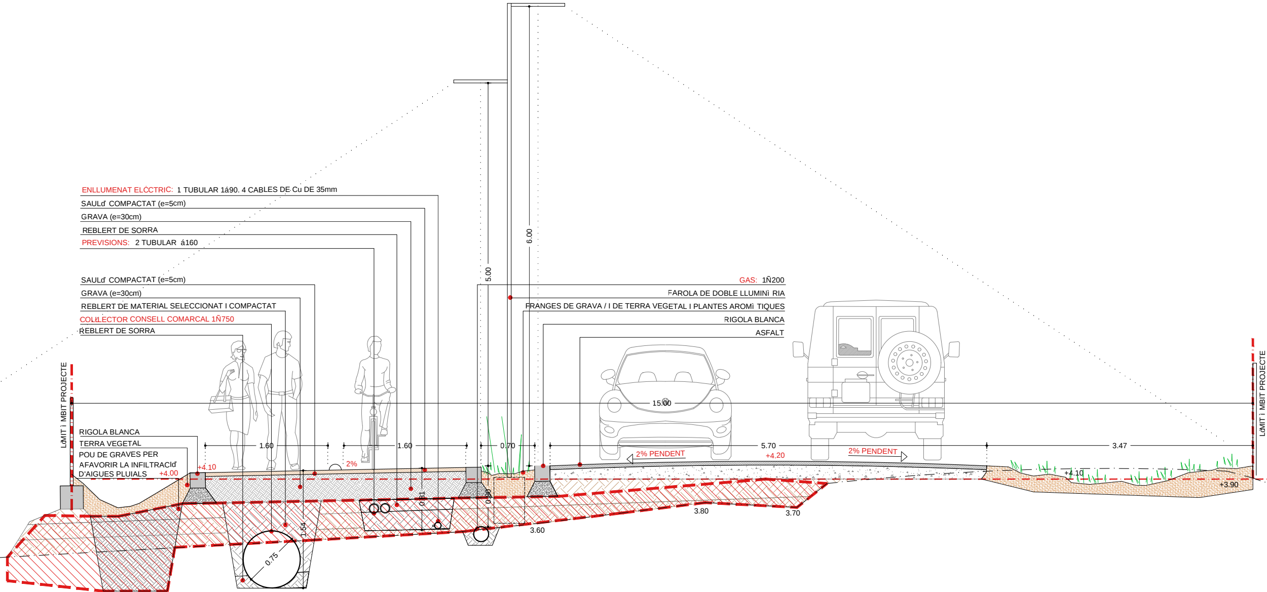
SECCIÓ 2. E:1/50
