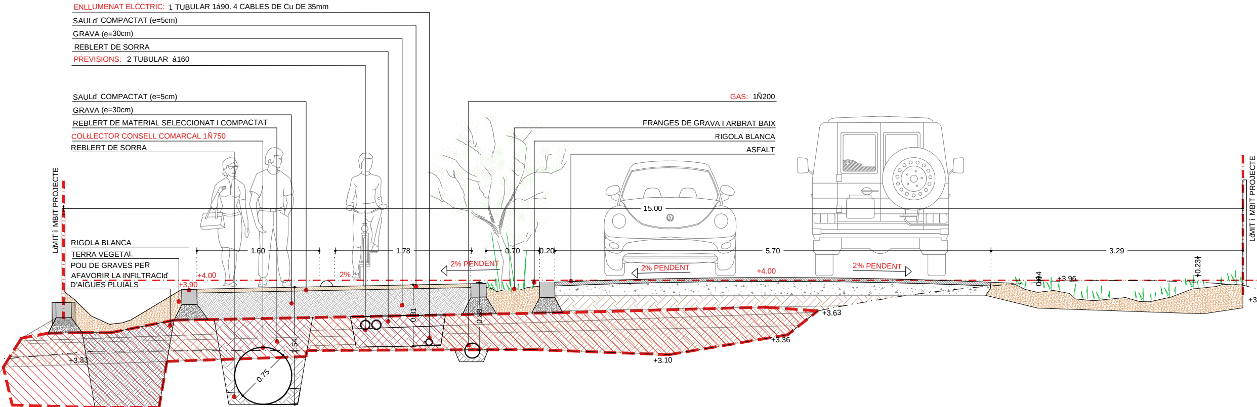
SECCIó 6. E:1/50
