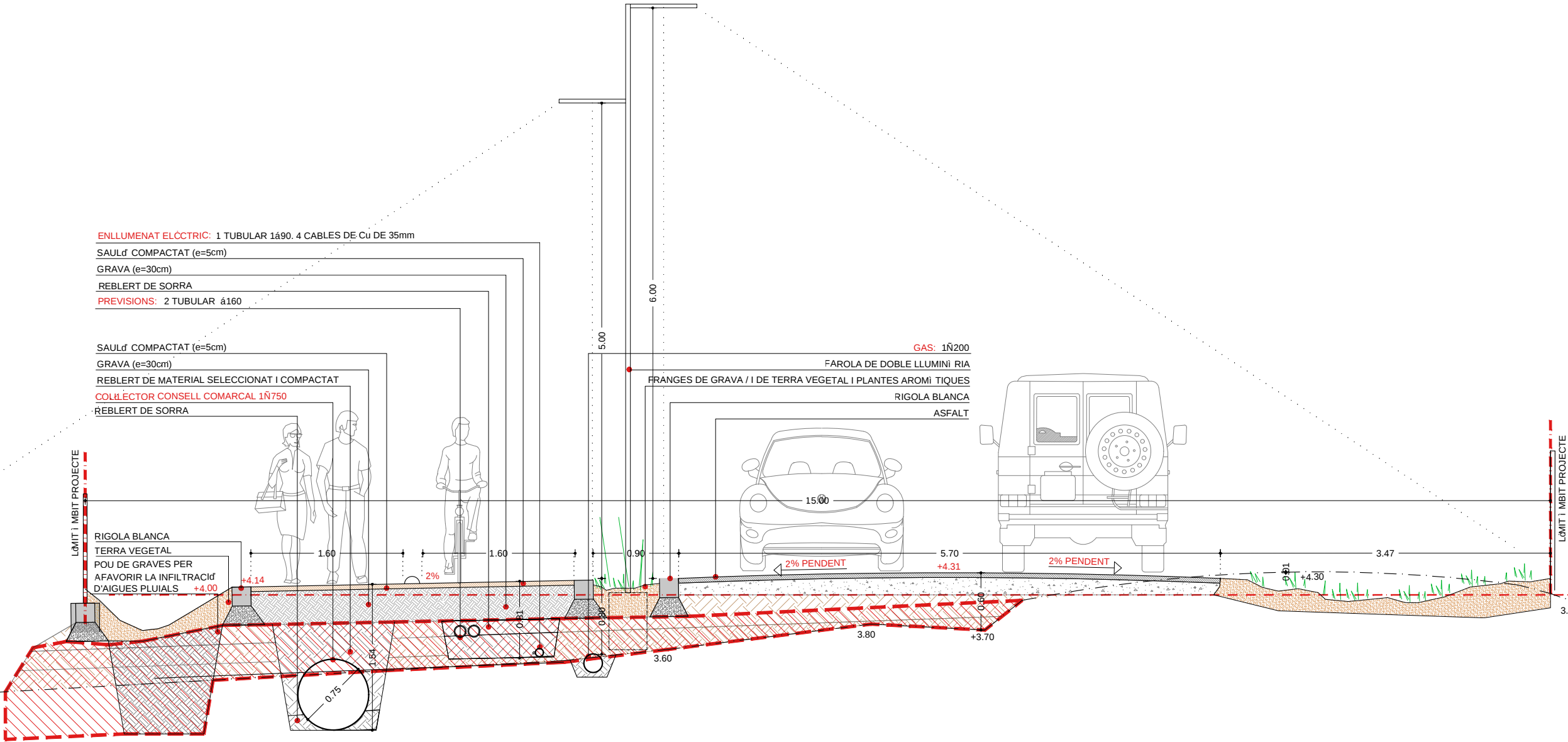
SECCIÓ 4. E:1/50
