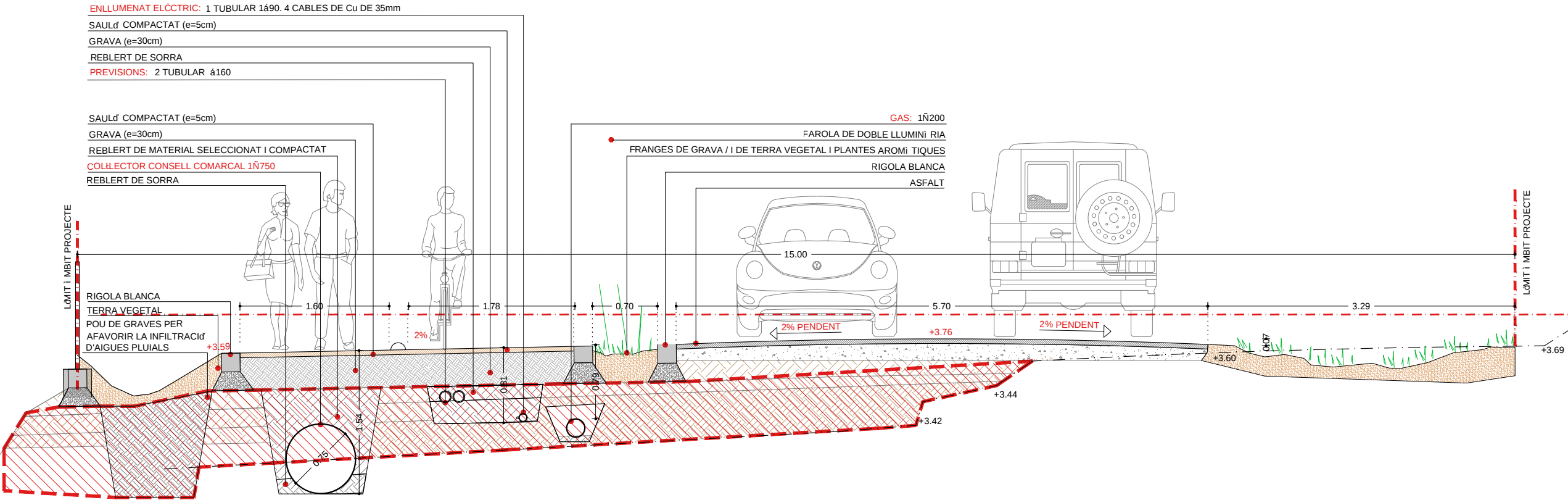
SECCIó 10. E:1/50
