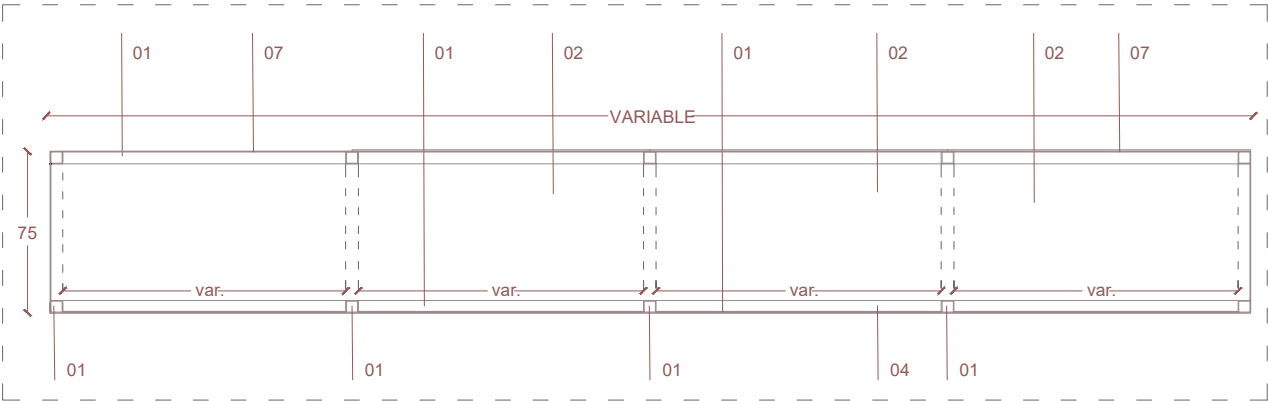
SECCIÓ HORIZONTAL PANEL TIPUS - VITRINA
