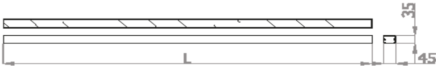
DIBUJOS TÉCNICOS LUMINARIA
