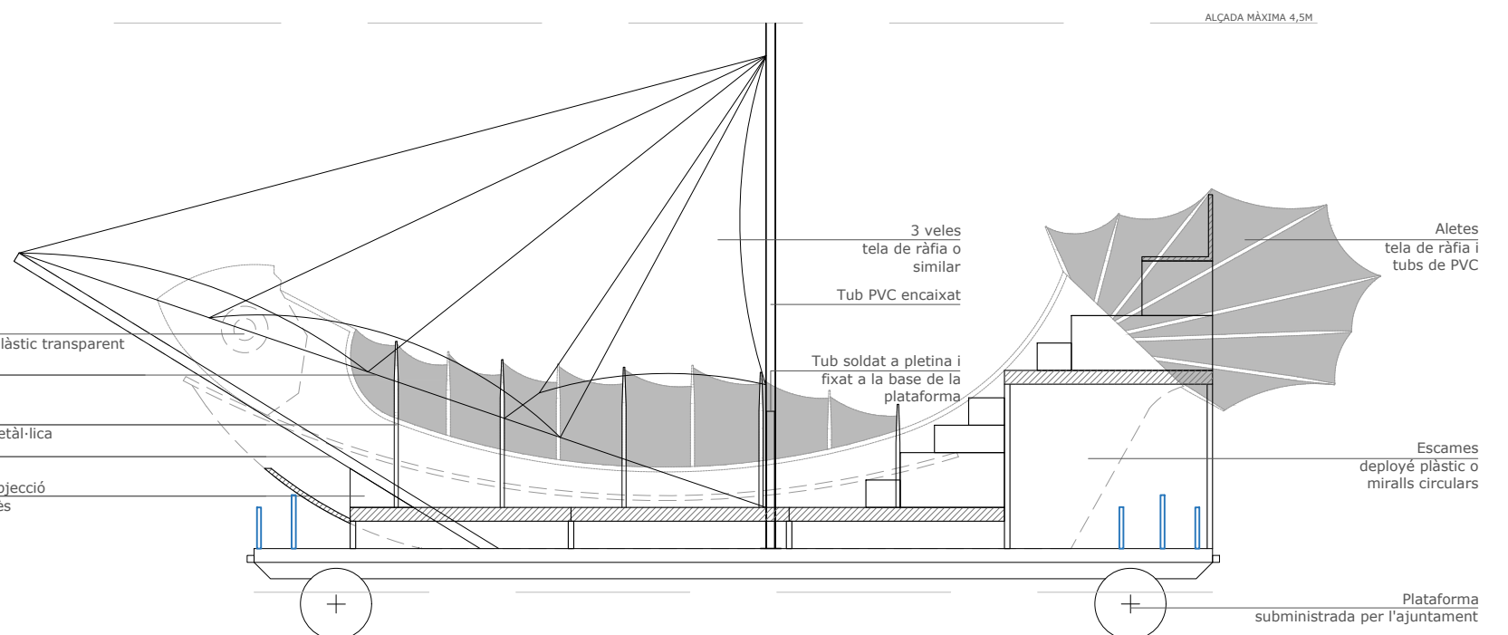
Secció longitudinal
