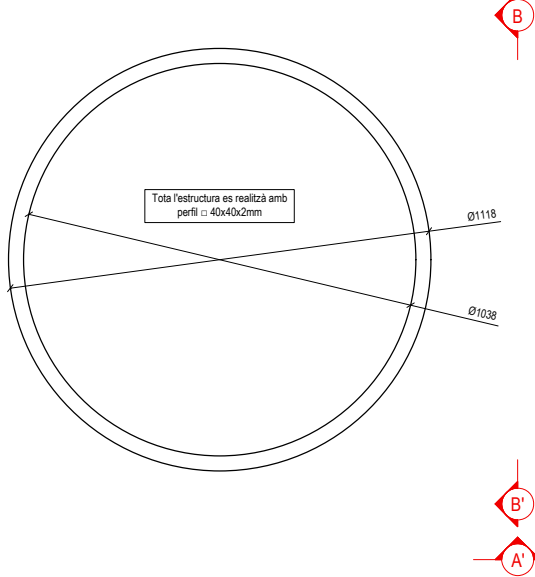
NIVELL 2
