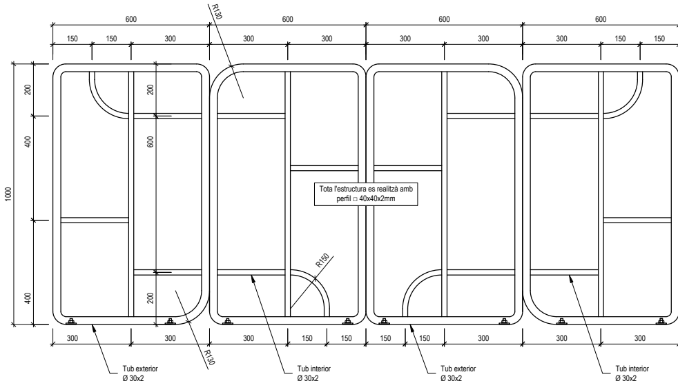
ALÇAT
