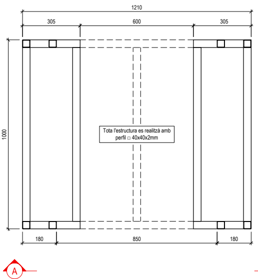
NIVELL 4
