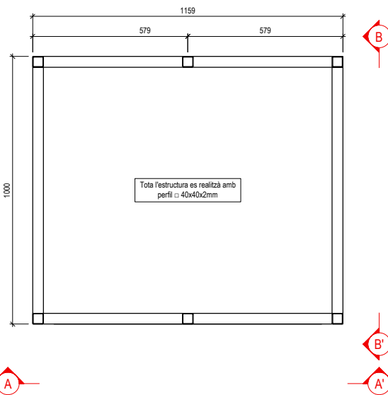
NIVELL 1
