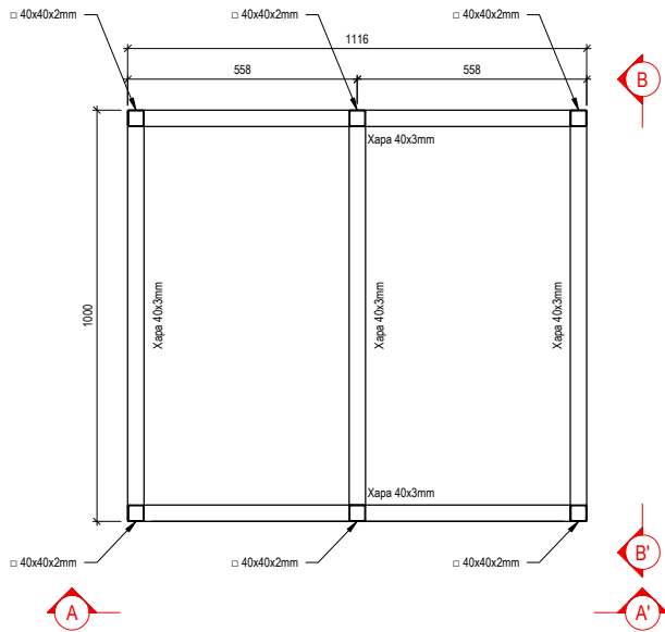
NIVELL 0
