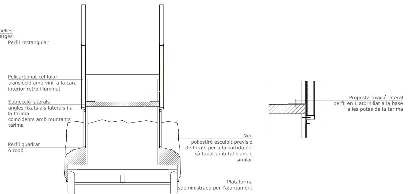
Secció transversal
