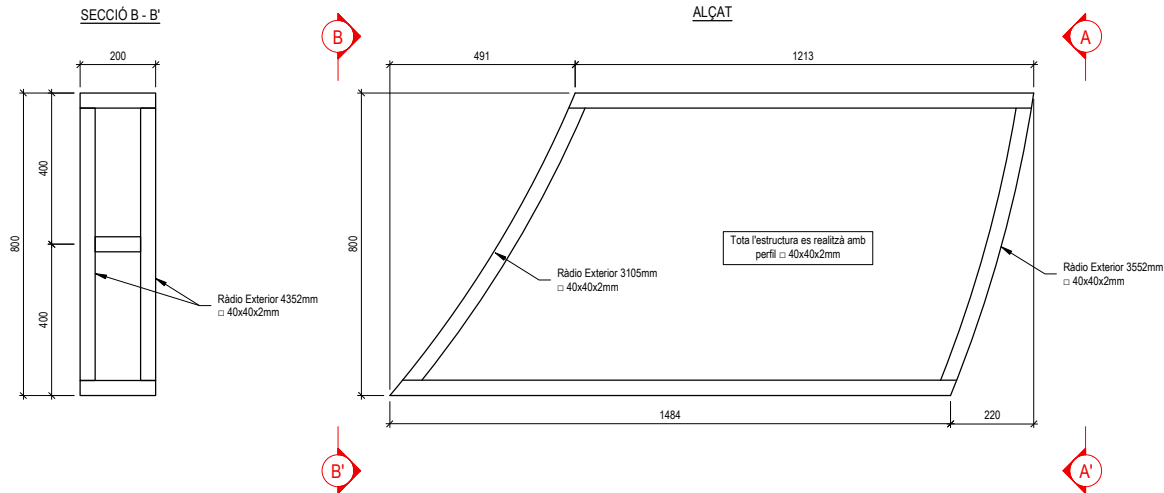
ELEMENT 2 (2 Uds.)
