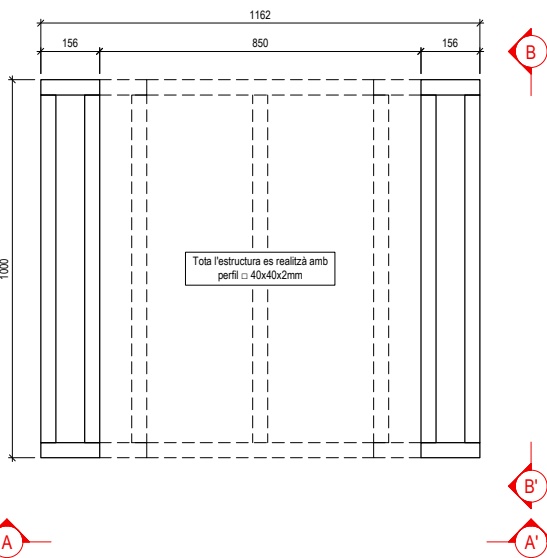
NIVELL 5
