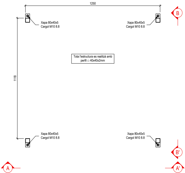
NIVELL 0
