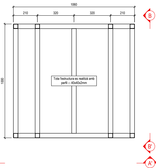
NIVELL 3
