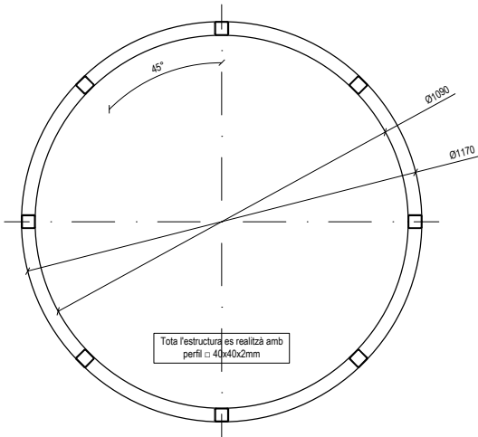
PLANTA
