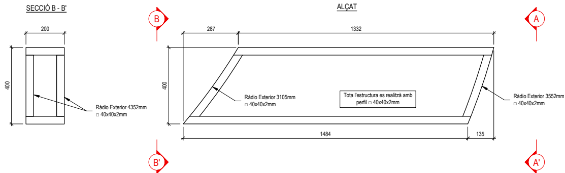
ELEMENT 5 (2 Uds.)
