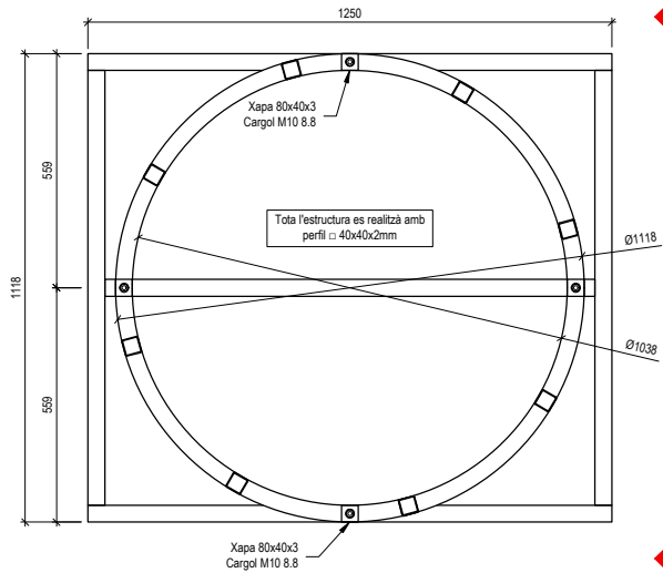
NIVELL 1
