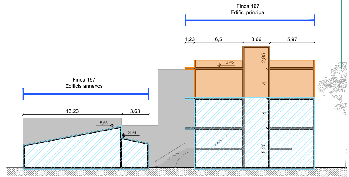
Secció B-B'
