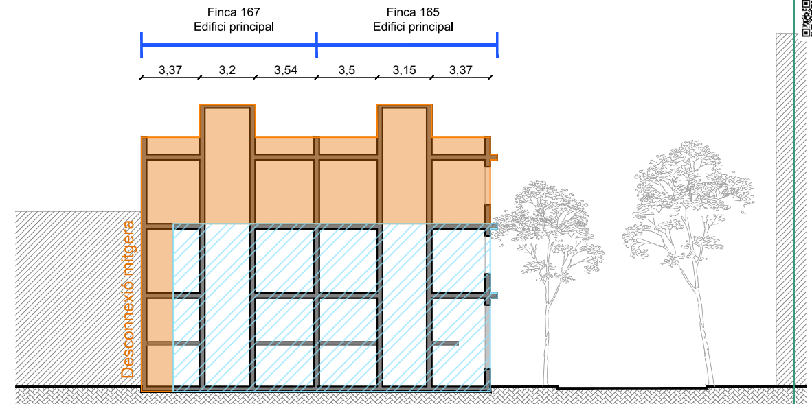
Secció A-A'
