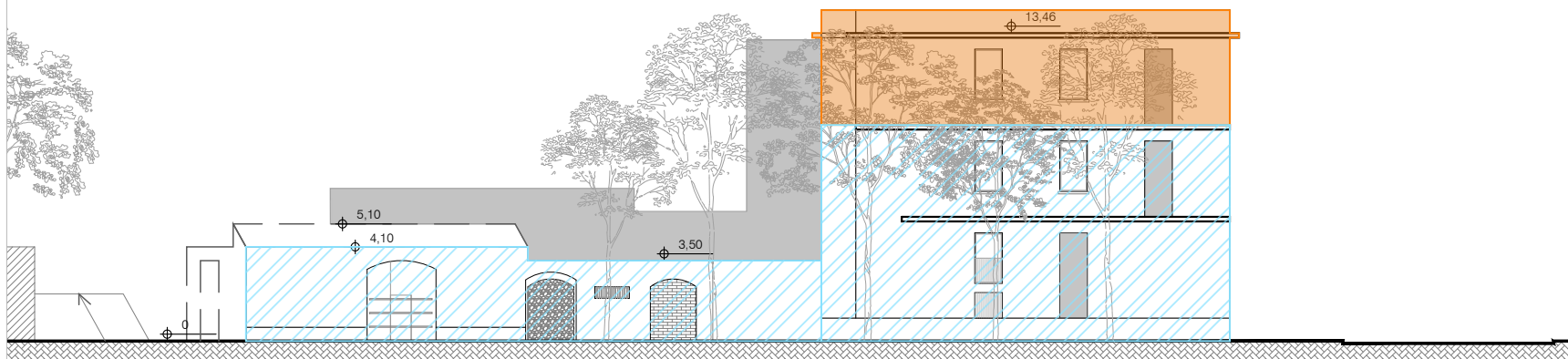
Alçat C/ de Portugal
