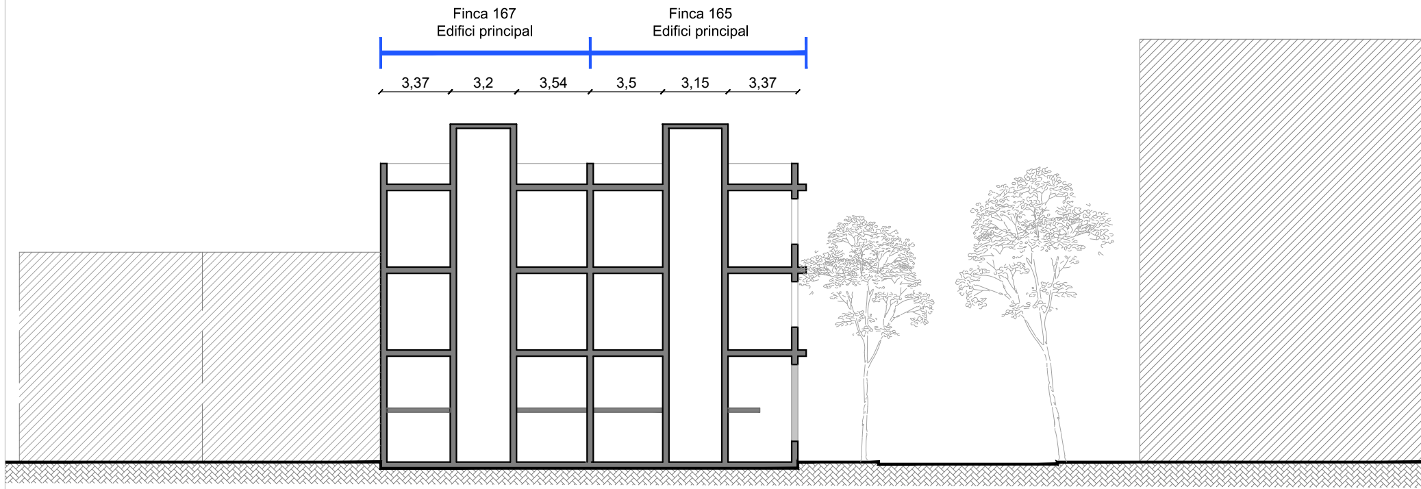
Secció A-A' e 1/250
