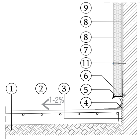
DETALL TROBAMENT MITGERA 2 E 1/10
