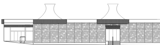
ALÇAT CC', CARRER DE FELIP II, E:1/250 0 5 10m
