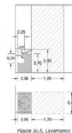
Figura 3c.5. Lavamanos
