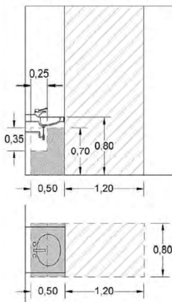
Figura 3c.5. Rentamans
