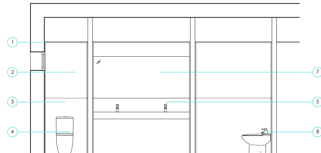
Alçat C-C'
