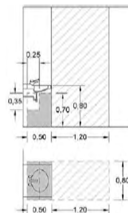
Figura 3c.5. Lavamanos
