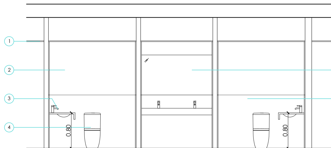
Alçat A-A'
