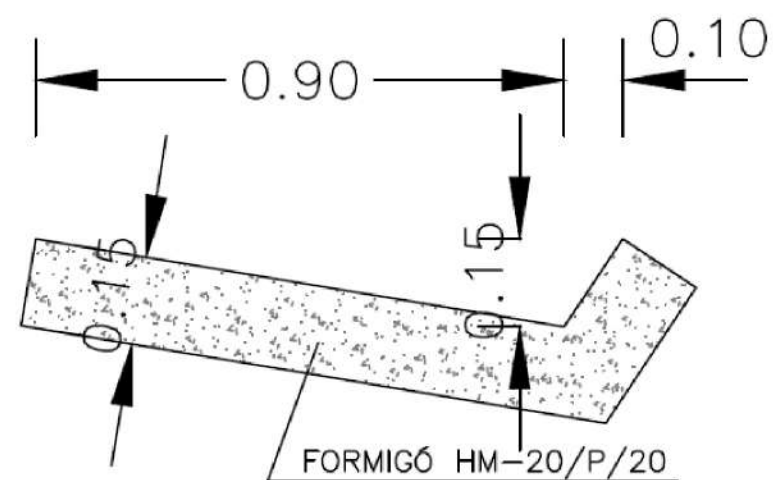
DETALL CUNETA REVESTIDA TIPUS TTR-10
