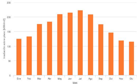
Irradiación mensual sobre plano fijo:
