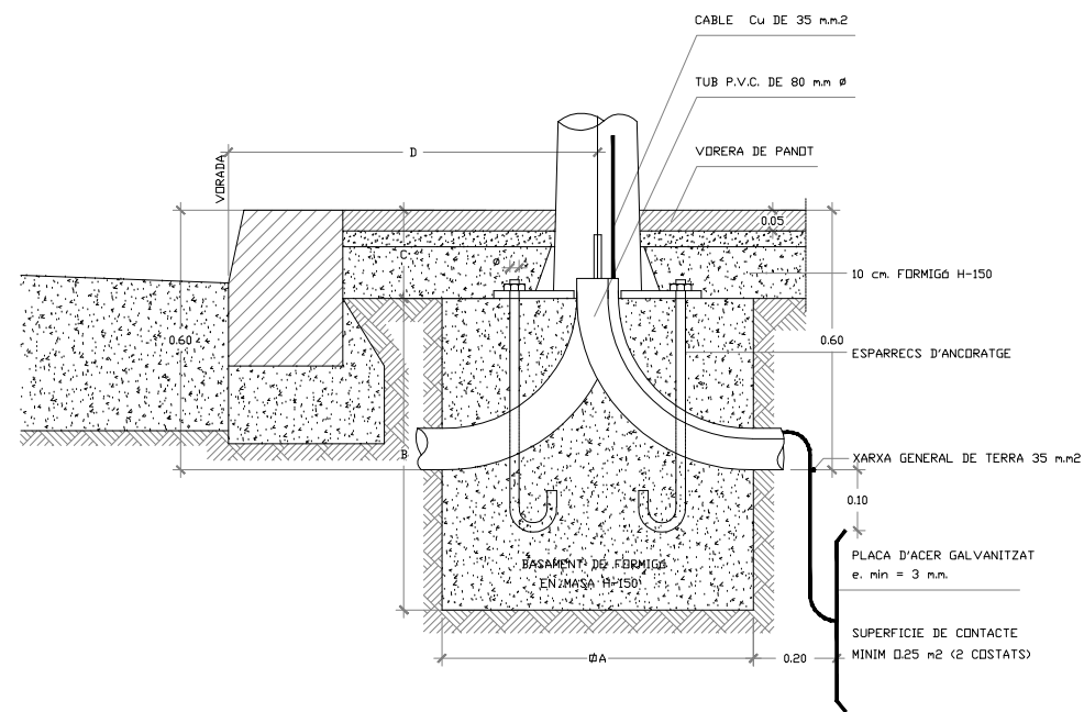
INSTAL·LACIÓ BACULS O COLUMNES E.1/10
