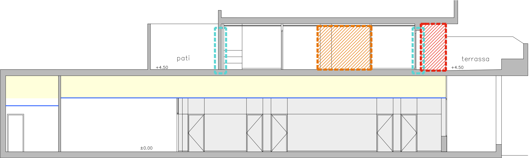
SECCIÓ 2
