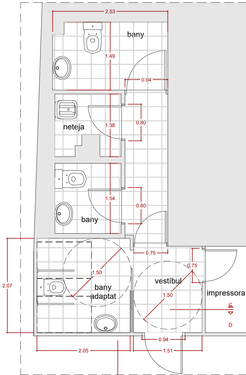
PLANTA
