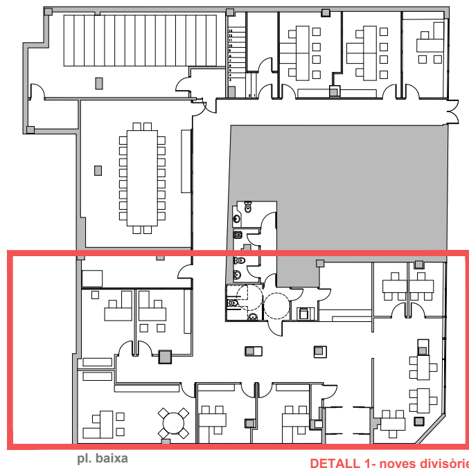
DETALL 1- noves divisòries
