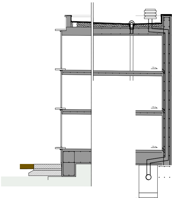
Secció tipus 1/50
