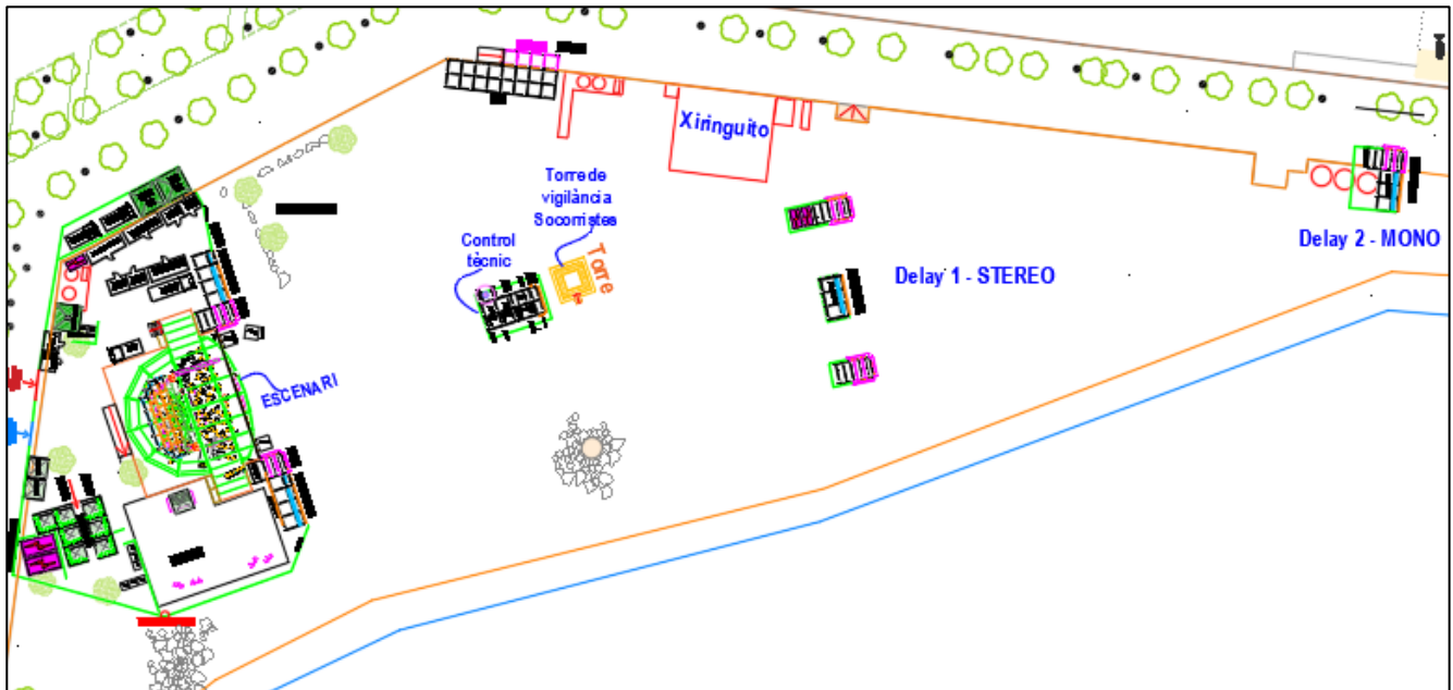
Plànol preliminar de la situació del muntatge
