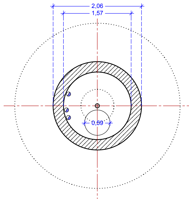
PLANTA TERCERA
