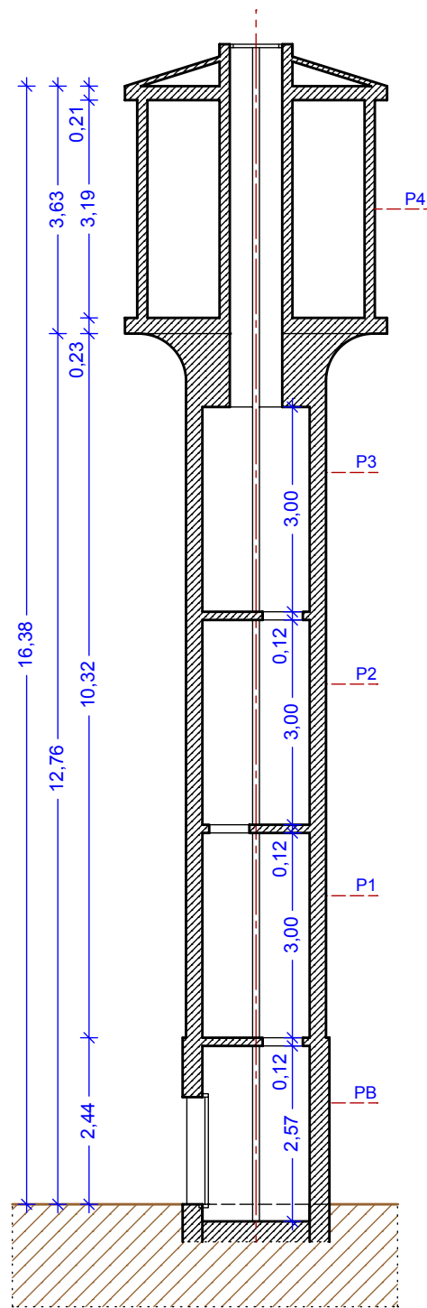
SECCIÓ (E: 1/100)
