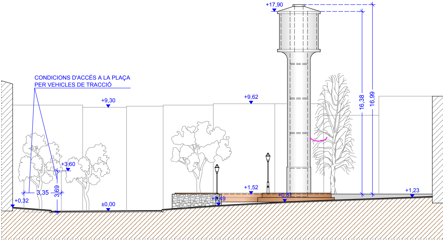
ALÇAT A-A'
