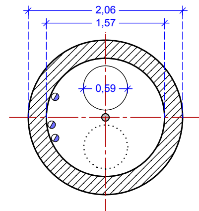
PLANTA SEGONA
