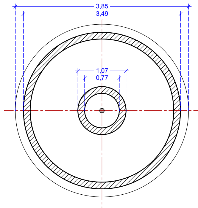
PLANTA QUARTA
