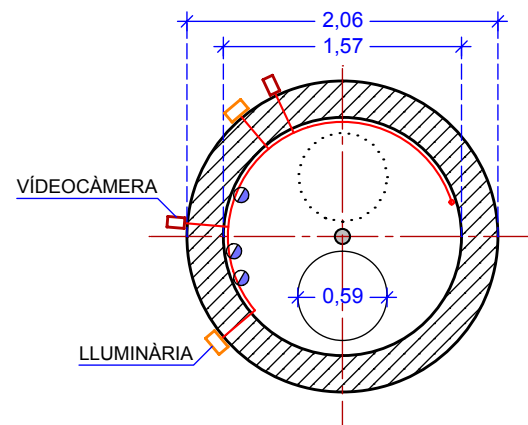
PLANTA PRIMERA
