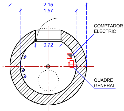
PLANTA BAIXA
