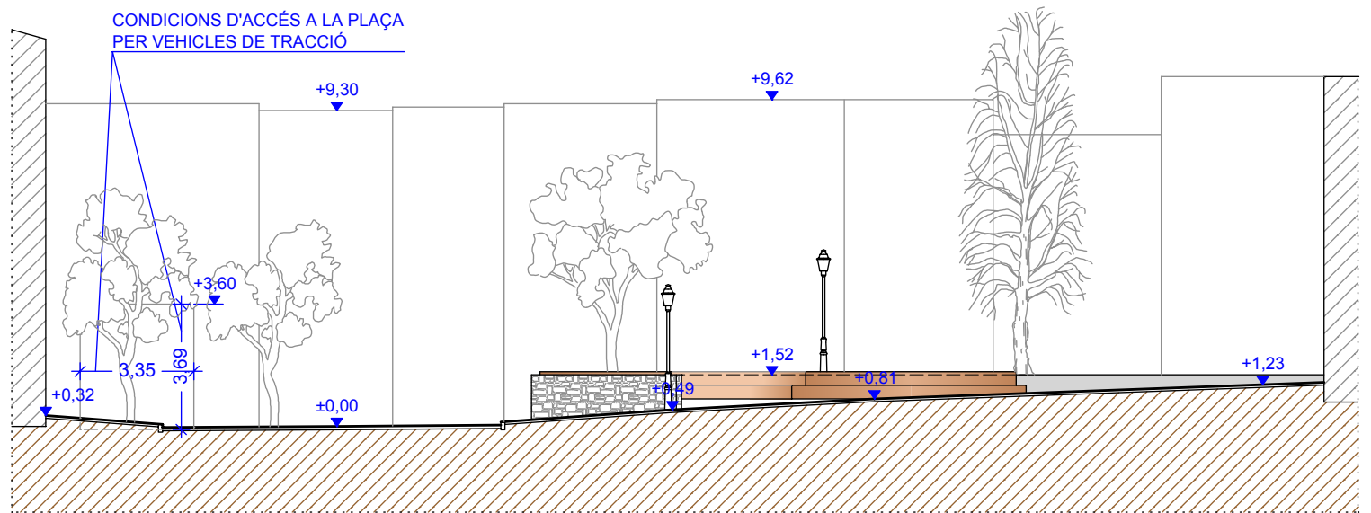
ALÇAT A-A'
