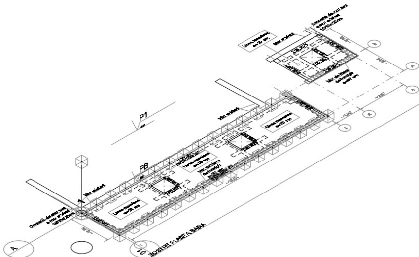
Imatge 5-1. Model de càlcul tridimensional
