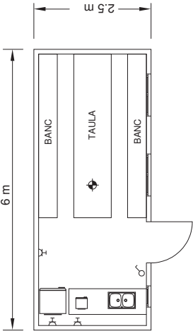
PLANTA
