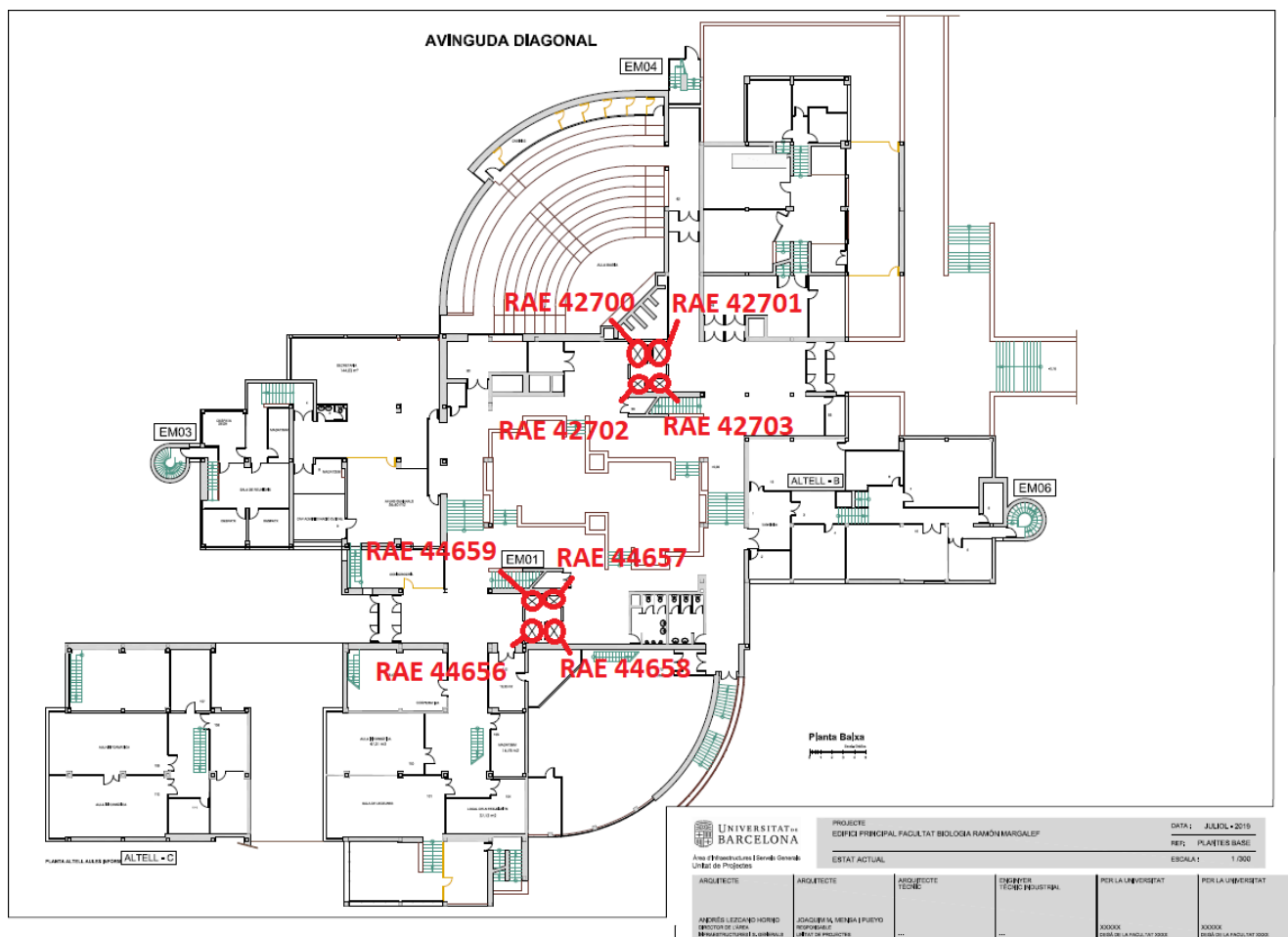
Plànol de distribució dels Ascensors de l'Edifici Margalef de la Facultat de Biologia (en Planta Baixa)
