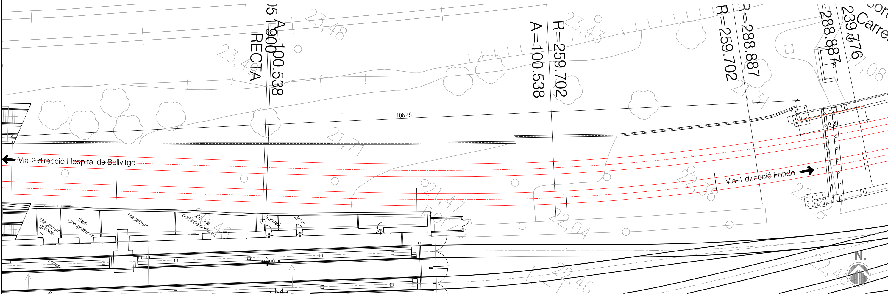
Planta Escala 1:300
