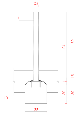
T01 SECCIÓ TANCA
