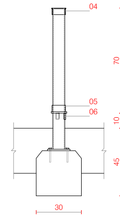
T02 SECCIÓ PORTA TANCA SABATA CORREGUDA FORMIGÓ HM-20/P/204 10 PUNTS SOLDATS 9 PUNTS ANCORATGE A SABATA AMB CARGOLS AMB FIXACIÓ DE TAC QUÍMIC 8 PLATINA 8MM GRUIX 7 TOPALLS SOLDATS AL TUB DE LA PORTA 6 ANELL SOLDAT A LA PLATINA INFERIOR DE LA PORTA DE 4MM GRUIX 5 ANELL SOLDAT A LA PLATINA SUPERIOR DE LA PORTA DE 4MM GRUIX 4 PORTA D'ENTRADA 3 SISTEMA DE TANCAMENT BASCULANT 2 TUB D'ACER GALVANITZAT Ø8CM I 1,5MM GRUIX AMB CANTELLS ARRODONITS I 8CM SEPARACIÓ 1
